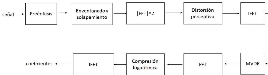
Figura 2. Diagrama funcional de la técnica PMVDR.
