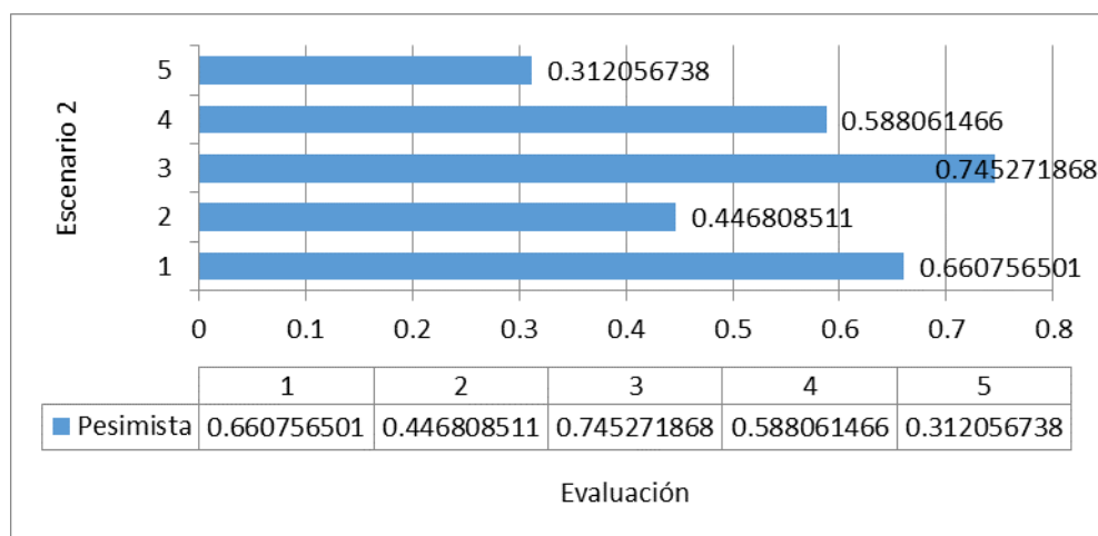
Fig. 6 - Comportamiento pesimista.
