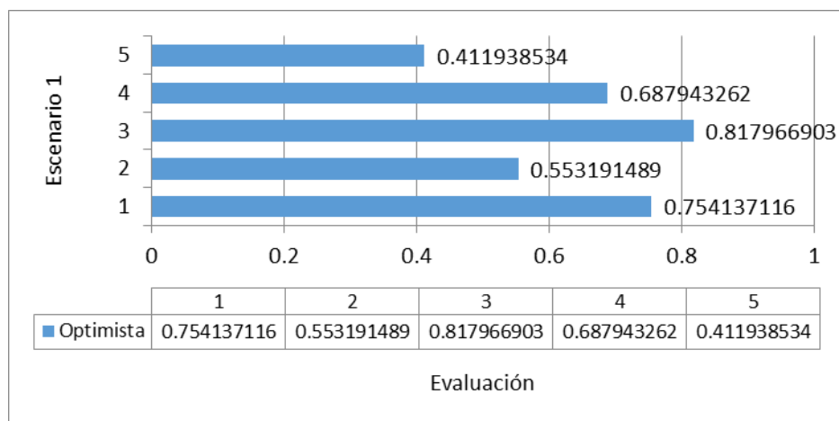
Fig. 5 - Comportamiento optimista.
