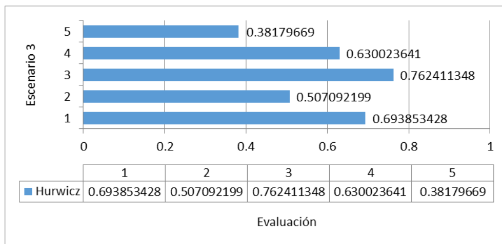
Fig. 7 - Comportamiento Hurwicz.
