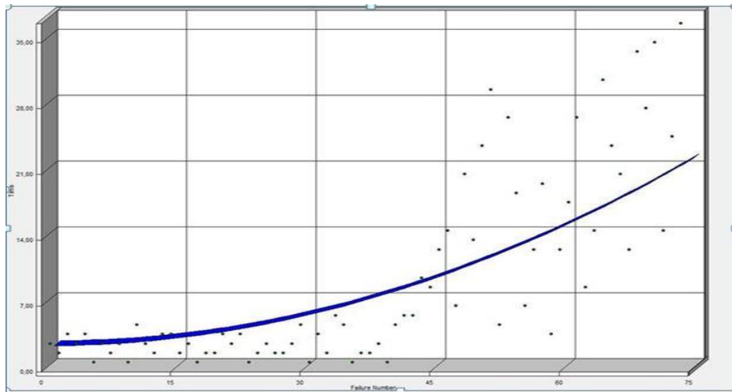
Fig. 1 - Resultados del método Littlewood-Verall en etapa implementación.
