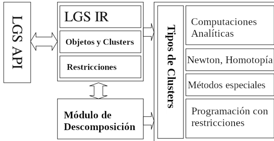
Fig. 6 - Arquitectura del solver LGS. Fuente:( Ershov et al., 2003 )
