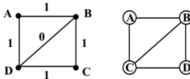
Fig. 5 - Un problema numéricamente infra-restringido (izquierda) y su grafo de restricciones asociado que si está bien restringido (derecha). Fuente: (Ait-Aoudia et al., 2009)
