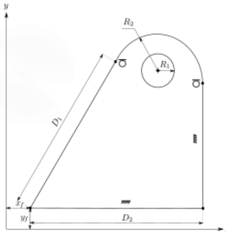
Fig. 2 - Perfil resultante de la aplicación de restricciones geométricas al croquiz de la Figura 1.
