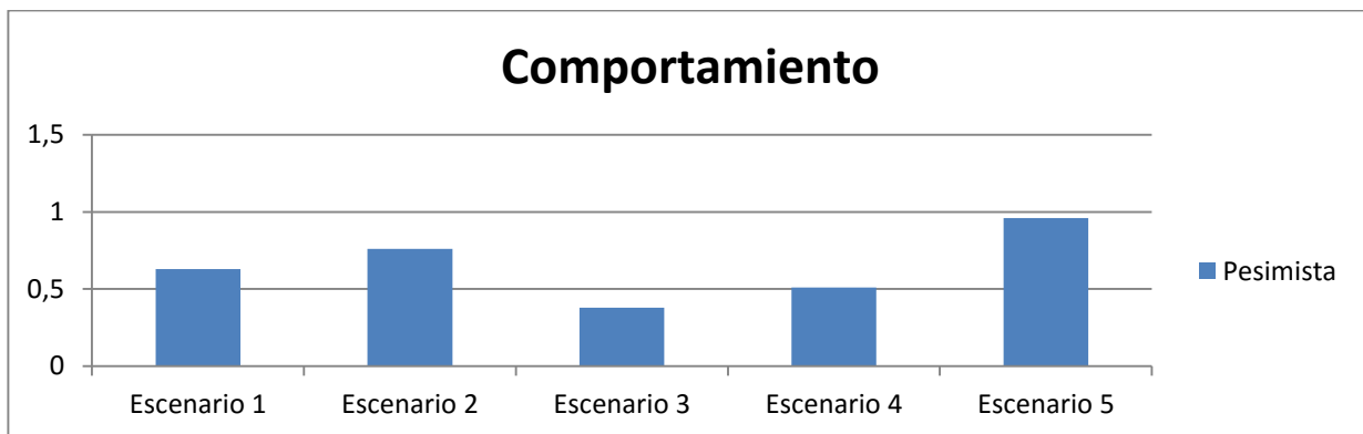
Fig. 8 - Comportamiento pesimista.
