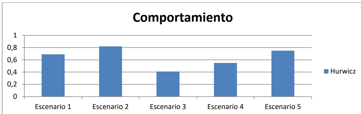
Fig. 6 - Comportamiento Hurwicz.
