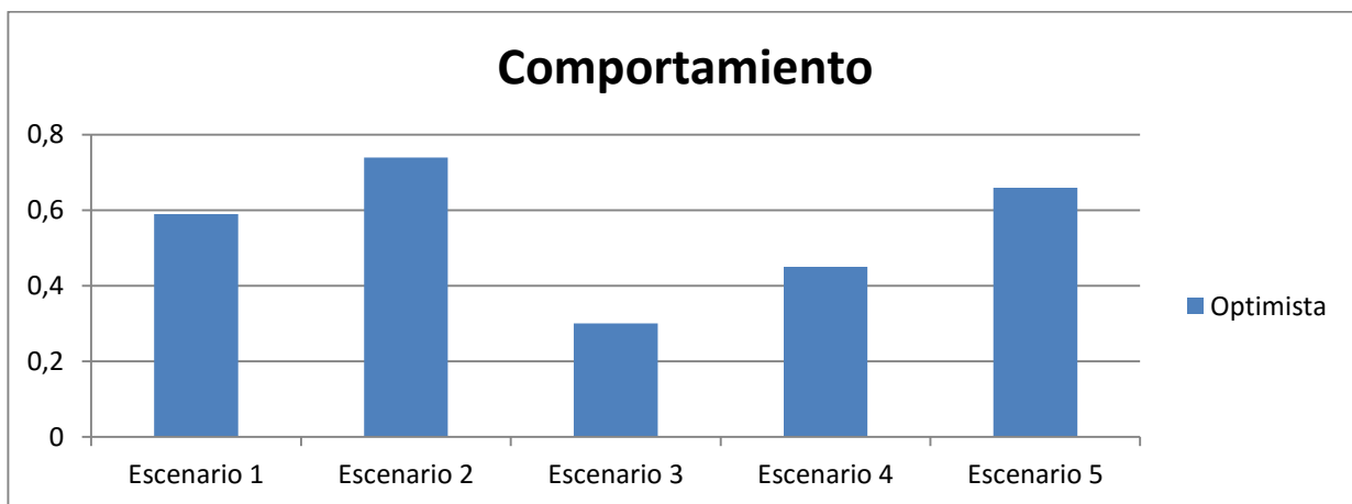
Fig. 7 - Comportamiento optimista.
