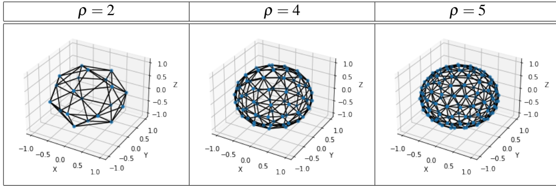
Fig. 1 - Distribución de puntos en una esfera unitaria para \rho \in \{2, 4, 5\} .
