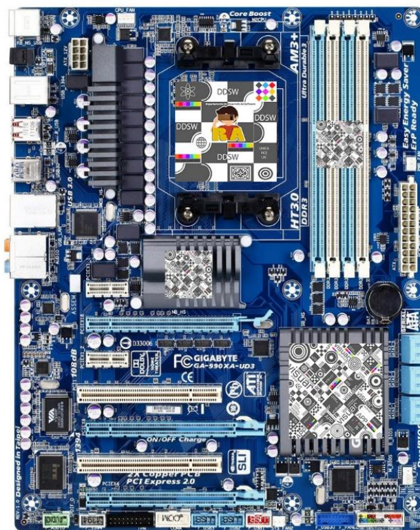
Fig. 2 - Motherboard para imprimir.
