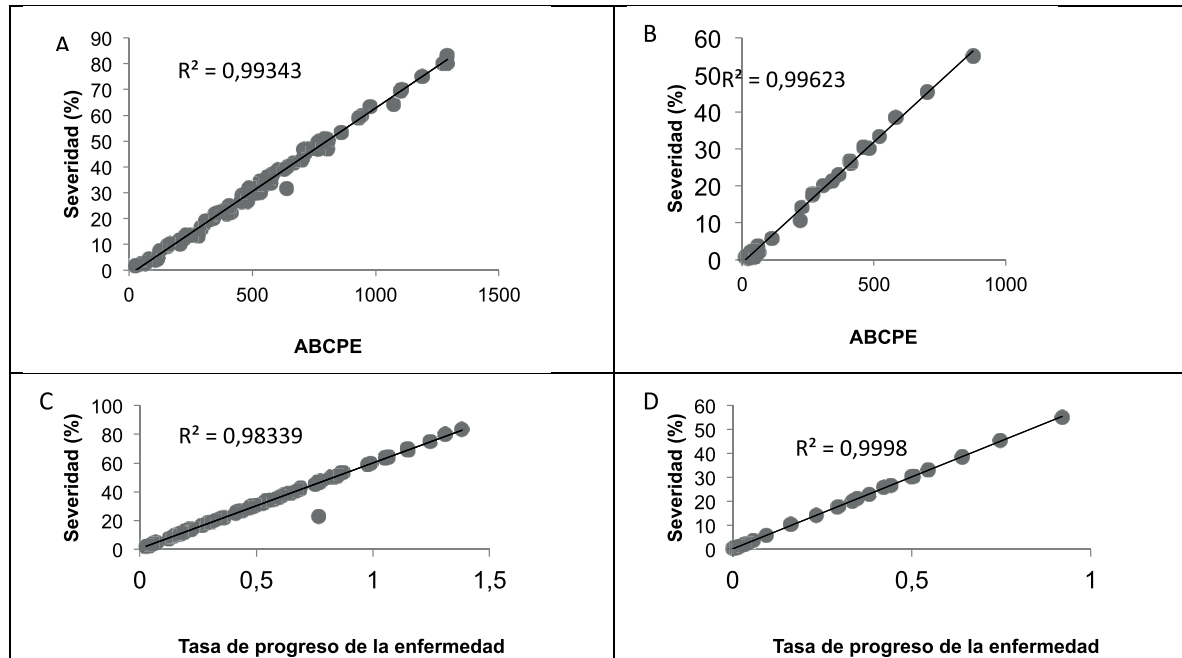
Figura 1. Relaciones entre la severidad de la antracnosis, en accesiones de ñame, a los 180 días, con el área bajo la curva de progreso ABCPE y la tasa de progreso de la enfermedad. A y C= D. alata ; B y D= D. rotundata ; ( p=0,01 )
