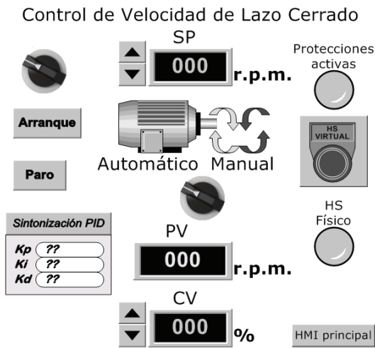
Figura 11. HMI para el control de velocidad de lazo cerrado
