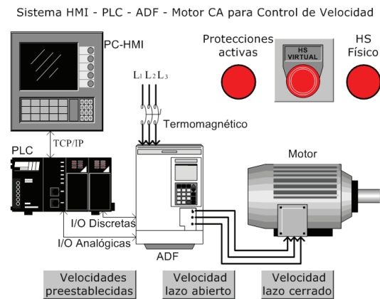
Figura 13. Protecciones del sistema activadas
