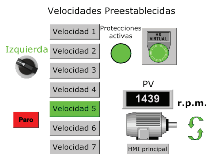
Figura 16. HMI velocidades preestablecidas, velocidad cinco
