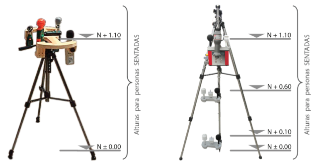
Figura 4. Izquierda: Instrumentos y alturas empleados en el estudio MER Cálido-húmedo . Derecha: Instrumentos y alturas empleados en el estudio ENS Semifrio-seco (Elaboración propia con base en ISO 10551, 1995 y ANSI/ASHRAE 55, 2017)
