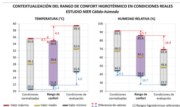
Figura 8. Relación del rango de confort higrotérmico con las condiciones normalizadas del periodo cálido y las condiciones de evaluación observadas en el estudio MER Cálido-húmedo (Elaboración propia)
