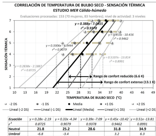
Figura 6. Correlación de la TBS y la ST con el método estadístico MIST para el periodo cálido del estudio MER Cálido-húmedo (Elaboración propia con base en Gómez et al. , 2007b)
