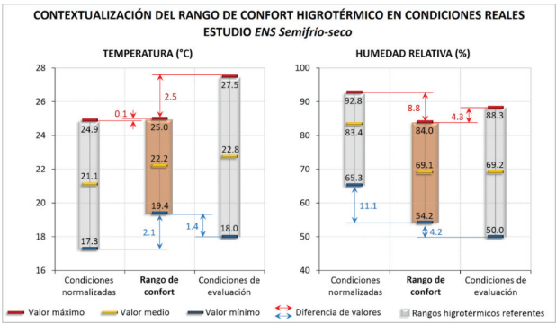
Figura 11. Relación del rango de confort higrotérmico con las condiciones normalizadas del periodo cálido y las condiciones de evaluación observadas en el estudio ENS Semifrio-seco (Elaboración propia)
