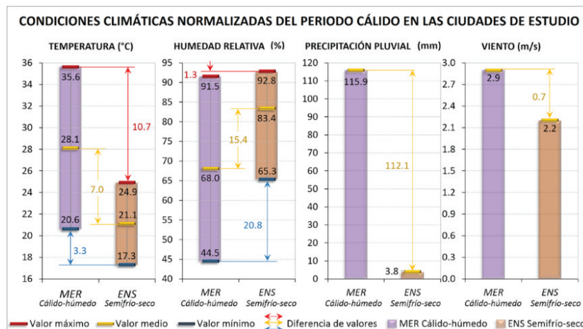
Figura 3. Comparativa de las condiciones térmicas, hídricas, hídricas y eólicas dadas durante el periodo cálido en los estudios MER cálido-húmedo (barra morada) y ENS semifrio-seco (barra café) (Elaboración propia con base en SMN-CONAGUA, 2019a y b)
