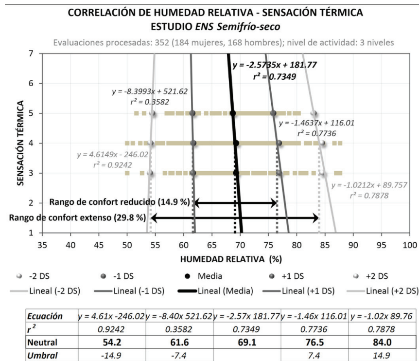
Figura 10. Correlación de la HR y la ST con el método estadístico MIST para el periodo cálido del estudio ENS Semifrío-seco (Elaboración propia con base en Gómez et al., 2007b)
