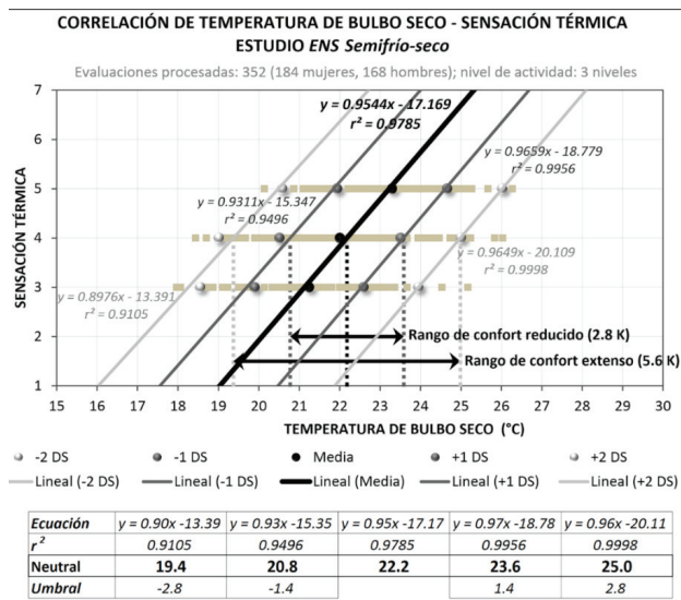
Figura 9. Correlación de la TBS y la ST con el método estadístico MIST para el periodo cálido del estudio ENS Semifrío-seco (Elaboración propia con base en Gómez et al., 2007b)
