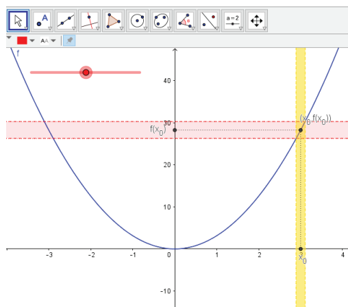
Figura 13. Archivo en GeoGebra para la actividad 2 del Taller 5.
