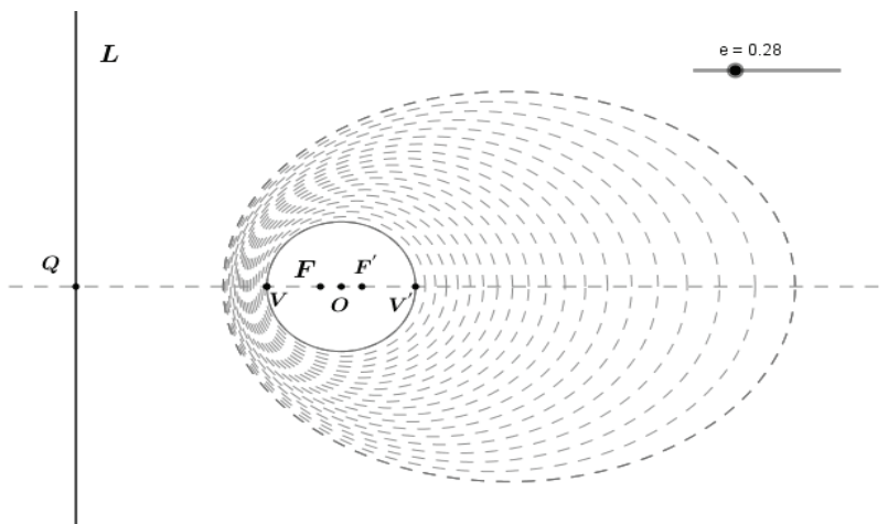
Figura 7. La elipse se colapsa en F cuando e \rightarrow 0 .
