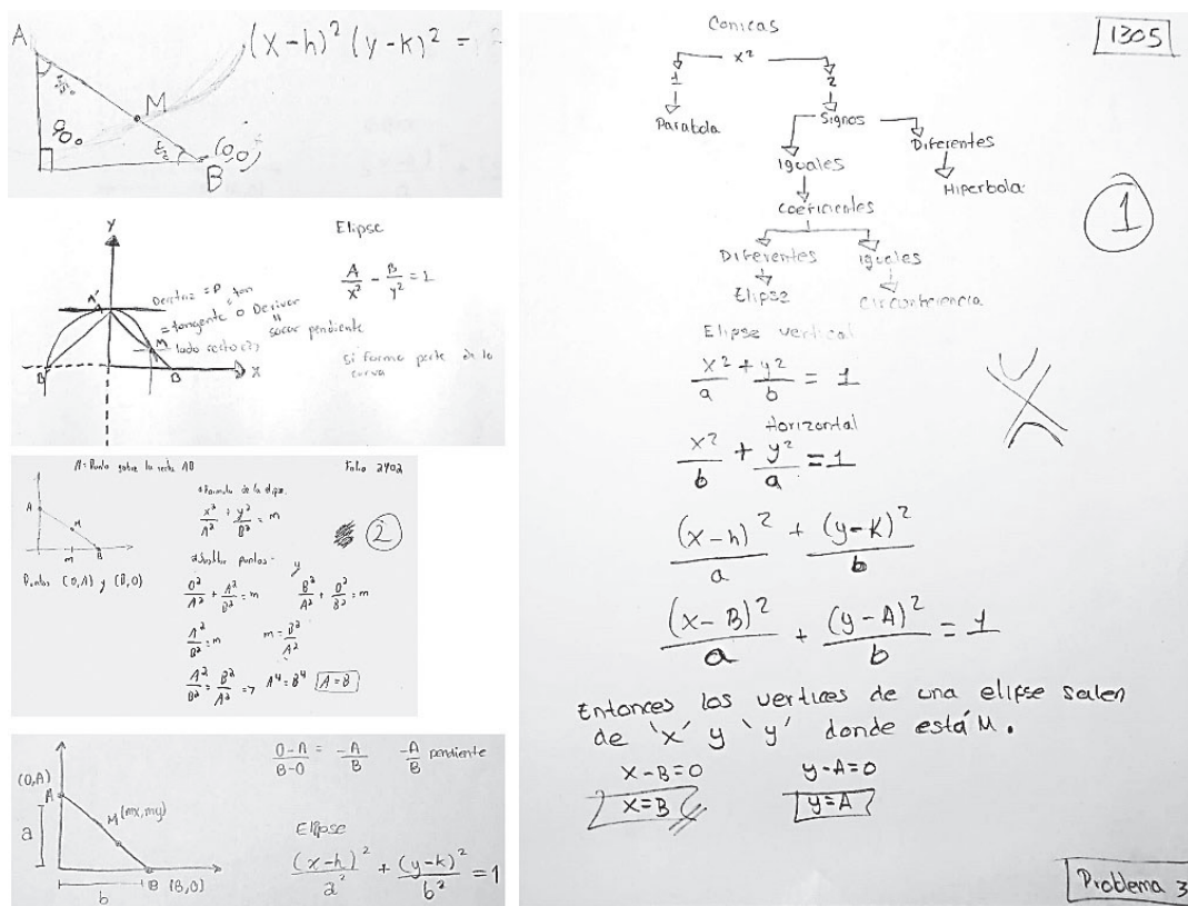
Figura 8. Búsqueda de conexión entre representaciones de la elipse.
