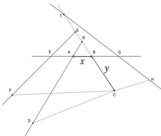
Figura 3. Sistema de referencia no ortogonal en la resolución del problema de Pappus . Los segmentos x e y, son lo que actualmente denominaríamos los ejes del sistema cartesiano. Fuente: Elaboración propia.
