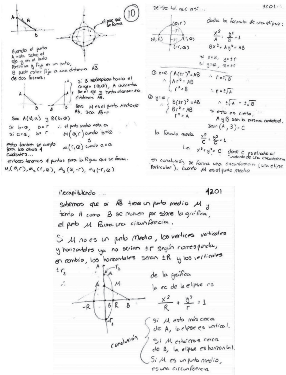
Figura 12. Relaciones visuales-algebraicas de la curva elipse.
