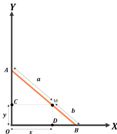
Figura 5. Elementos geométricos necesarios para el abordaje de la situación.
