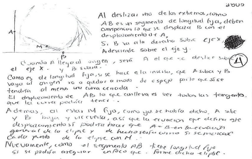
Figura 9. Deducción particular del comportamiento de los extremos A y B del segmento.
