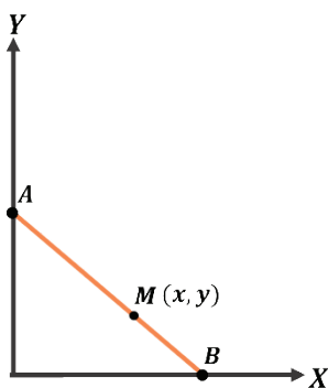
Figura 4. Segmento AB con un punto fijo M , sobre los ejes cartesianos.
