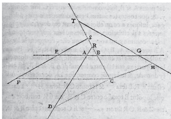
Figura 2. Problema de locus resuelto por Descartes.
