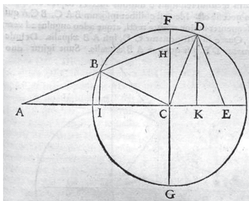
Figura 1. Problema resuelto por Viète relativo a la trisección del ángulo.
