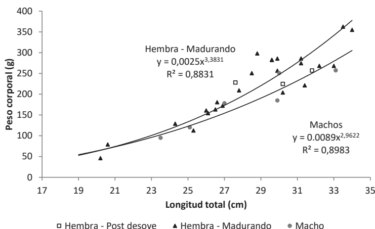
FIGURA 3. Relación longitud total–Peso de Eremophilus mutisii .
