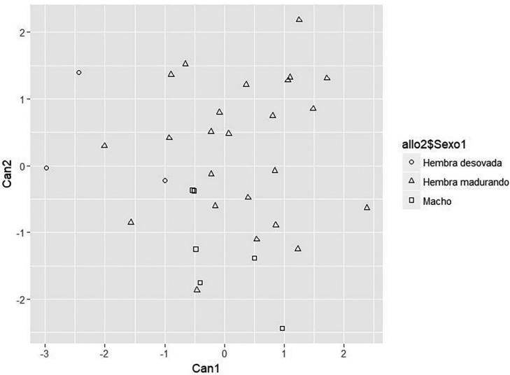
FIGURA 2. Plano de dispersión de las funciones discriminantes para diferentes condiciones reproductivas de Eremophilus mutisii .
