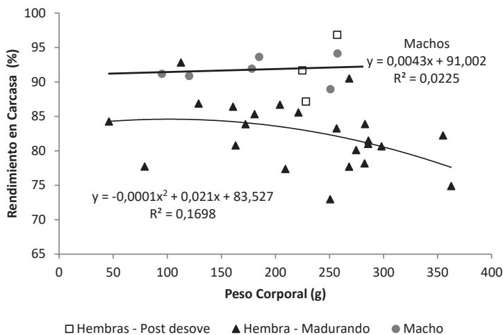
FIGURA 5. Relación peso corporal – rendimiento en carcasa de Eremophilus mutisii .
