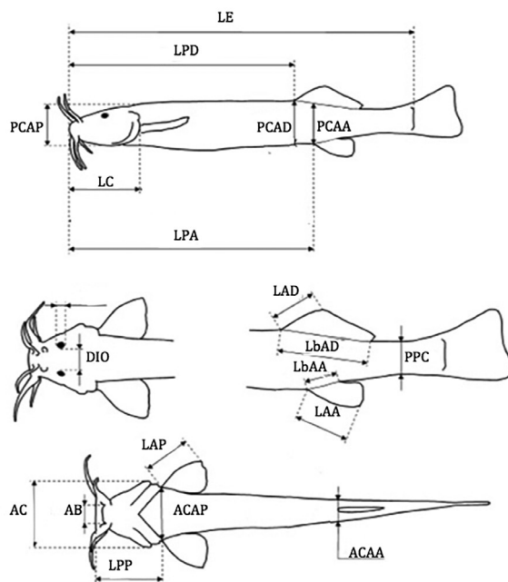
FIGURA 1. Medidas corporales tomadas en Eremophilus mutisii (Modificado de Barriga y Battini 2009).
