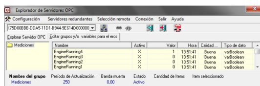
Figure 7. Registers reading of the Hyundai groups through OPC Lecturas de registros de los grupos Hyundai a través de OPC
