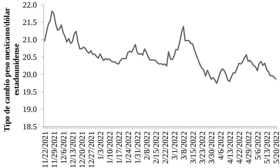
Gráfica 2 Tipo de cambio diario entre el peso mexicano y el dólar norteamericano 22 de noviembre de 2021 a 20 de mayo de 2022 (126 observaciones)
