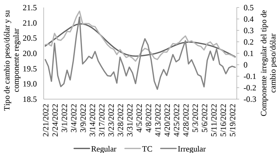
Gráfica 6 Componentes de la serie Tipo de Cambio (3 meses)
