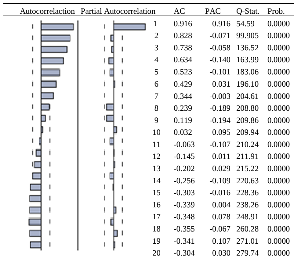
Gráfica 3 Correlograma del tipo de cambio para 62 observaciones
