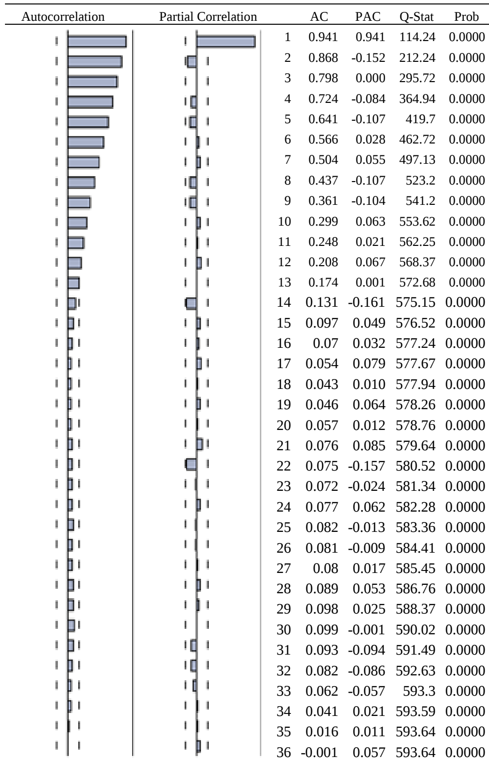
Gráfica 4 Correlograma del tipo de cambio para 126 observaciones
