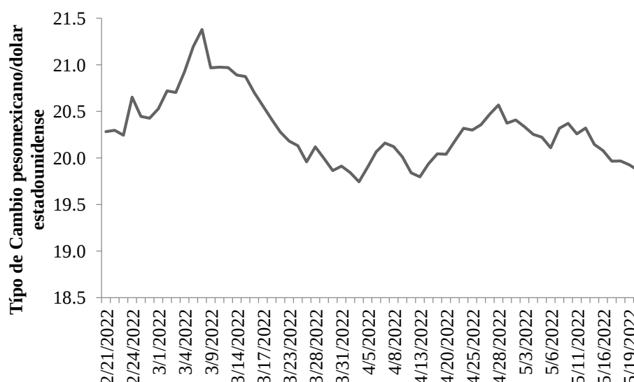
Gráfica 1 Tipo de cambio diario entre el peso mexicano y el dólar norteamericano, 21 de febrero a 20 de mayo de 2022 (62 observaciones)
