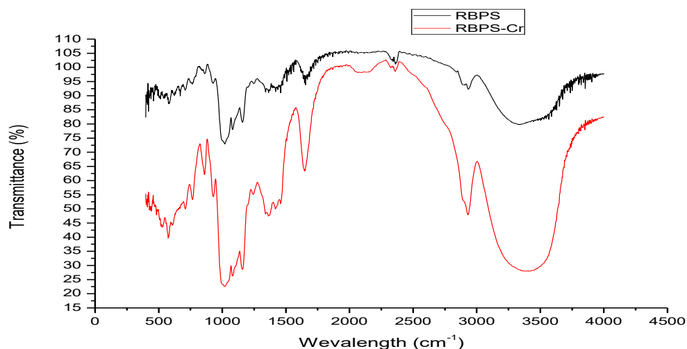
Fig. 1. Espectro FTIR para la biomasa residual de almidón de plátano (SBPS) antes y después de la adsorción de Cr (VI) (SBPS-Cr).
