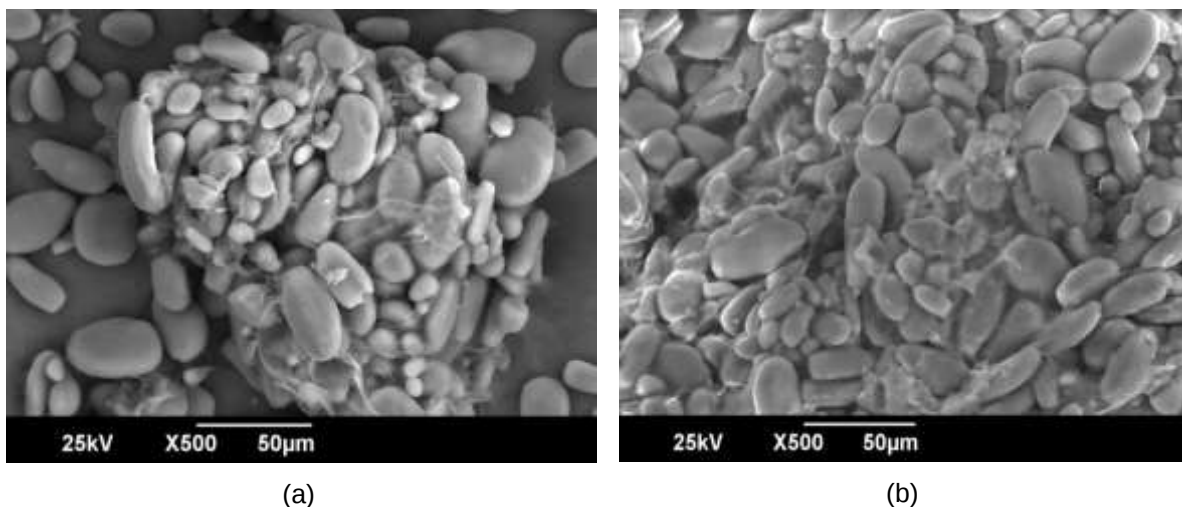
Fig. 2. Imagen SEM de la biomasa residual de plátano antes de la adsorción (a) y después de la remoción de Cr (VI) (b)
