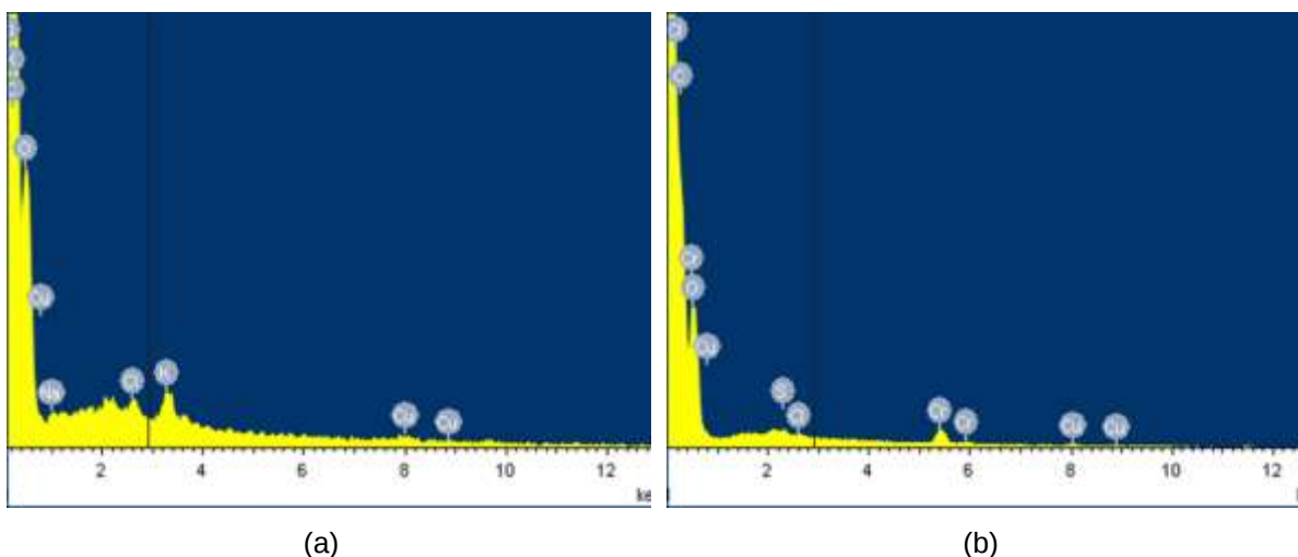
Fig. 3. Análisis EDS de la biomasa residual de plátano (a) antes de la adsorción y (b) después de la remoción de Cr (VI).
