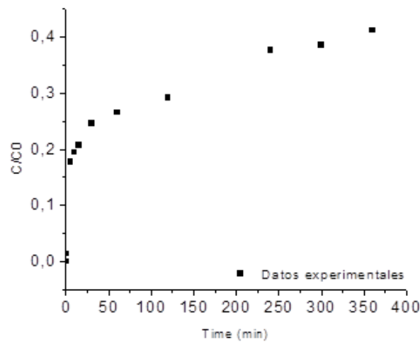
Fig. 6. Curva de avance de la adsorción de Cr (VI).
