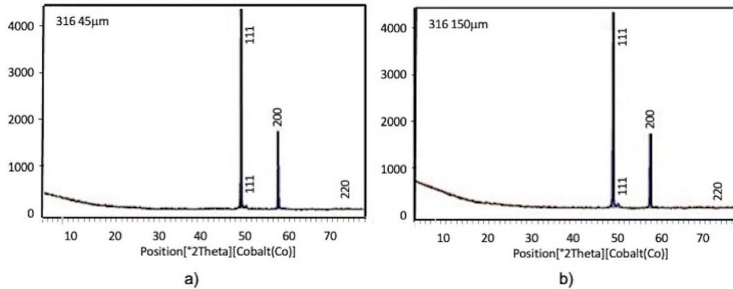
Fig. 1. AISI 316 steel powder diffractogram a) 45µm; b) 150µm.
