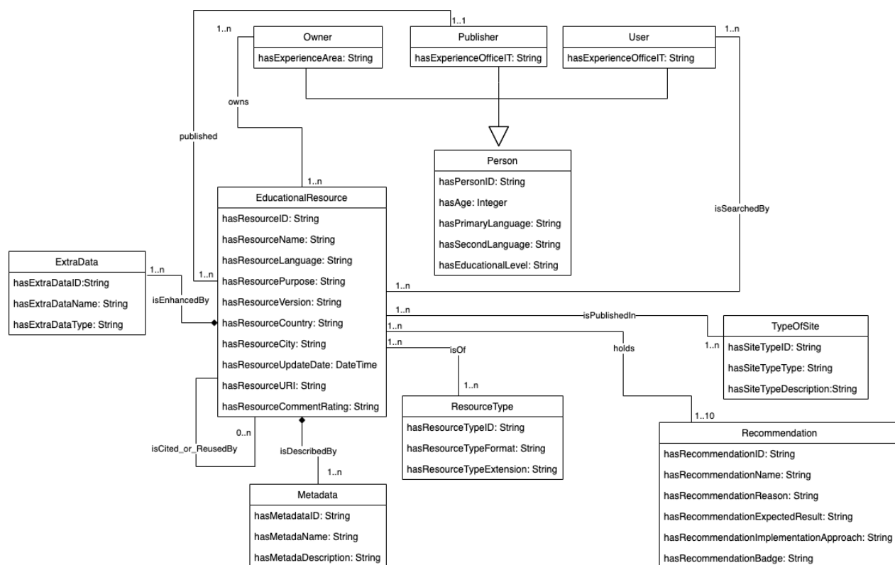
Figura 4. Diseño general de la ontología
