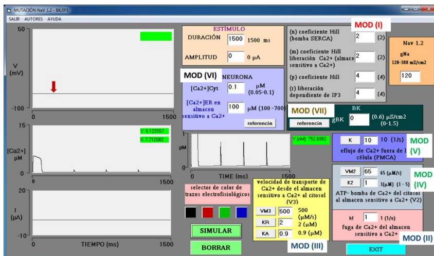
Figura 1. Interfaz del simulador EpiNav. Se muestran los módulos de entrada de datos que controlan las oscilaciones de \text{Ca}^{2+} citosólico (MOD I al MOD VI). Los osciloscopios centrales registran estas oscilaciones: una salida abrupta de \text{Ca}^{2+} con una amplitud de \sim 5 \mu\text{M} seguida de oscilaciones de \sim 752 \text{ nM} . En esta neurona no exciten canales BK, g_{\text{BK}} = 0 \text{ mS/cm}^2 (MOD VII). El osciloscopio superior muestra el registro intracelular de la neurona (flecha roja), neurona silente. El osciloscopio inferior indica que no se estimuló eléctricamente a la neurona.
