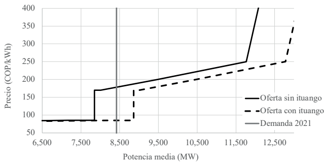
Figura 1. Curva de oferta del sistema con y sin Ituango
