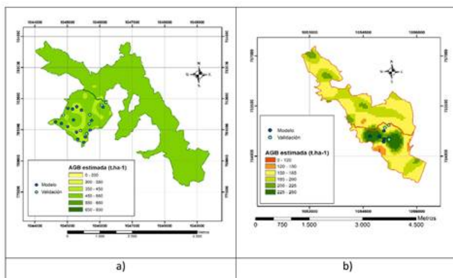
Figura 4 Distribución de AGB estimada: A) E. grandis ; B) P. spp .
