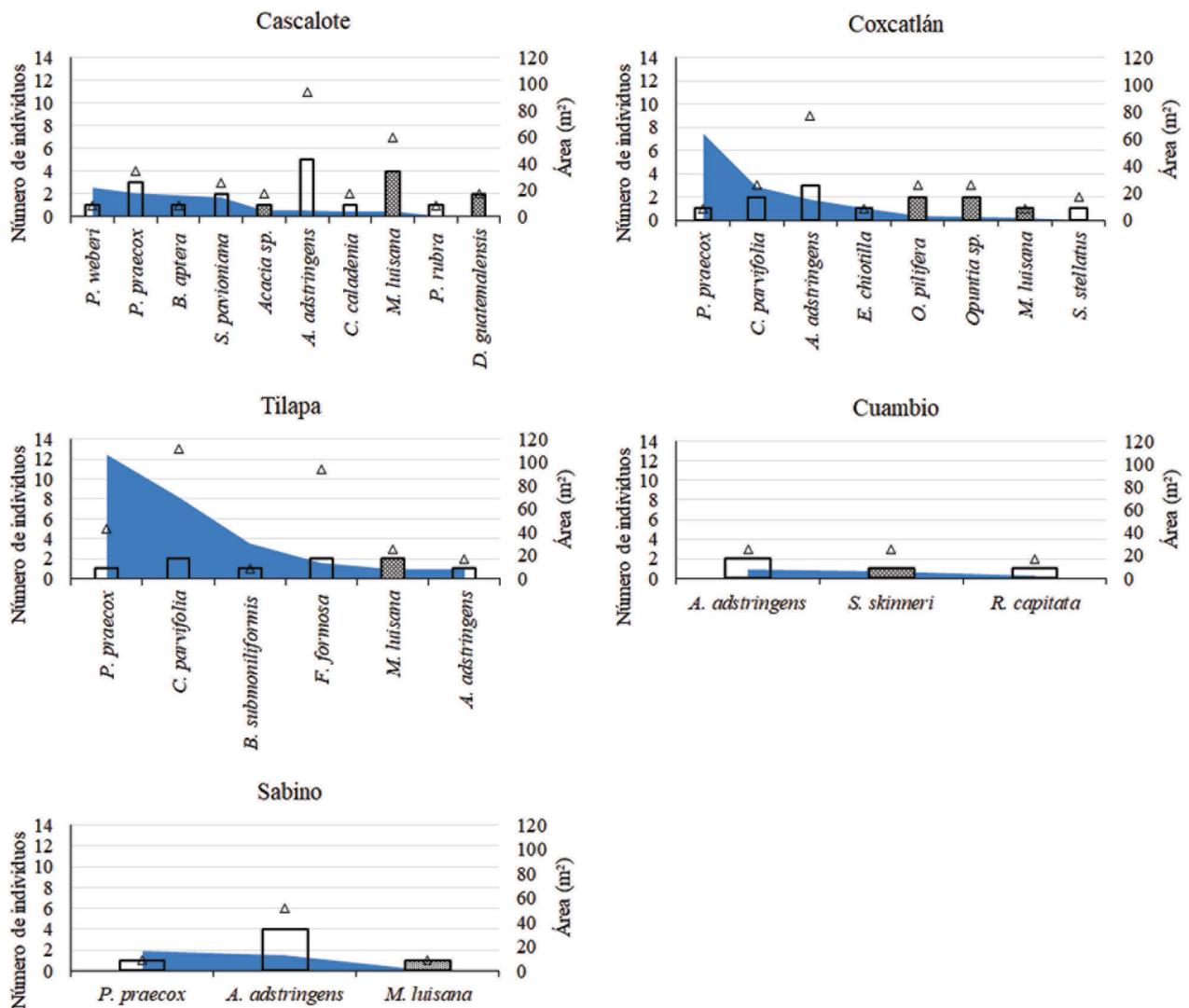
Figura 2. Relación entre el número de individuos asociados de A. adstringens (triángulos), el tamaño de la copa (área azul) y el número de plantas adultas (barras) en los sitios de estudio. Las barras vacías indican especies arbóreas y las barras llenas especies arbustivas. El tamaño de la copa representa el área promedio de las plantas adultas.
