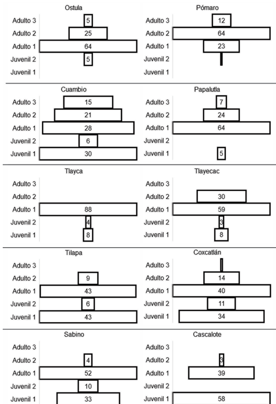
Figura 1. Estructuras de edad de A. adstringens en los sitios de estudio. Los números representan el porcentaje de individuos en cada categoría de edad.
