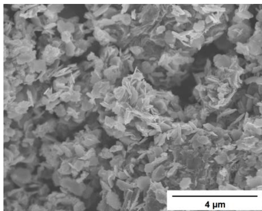
Figura N° 11. Micrografías SEM. SnS 2 -24H
