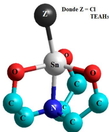
Figura N° 5. Complejo estannatrano (autoría propia)
