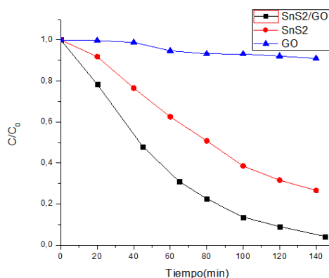
Figura N° 12. Variación de la concentración relativa (C/C 0 ) en función del tiempo en los procesos de degradación fotocatalítica.
