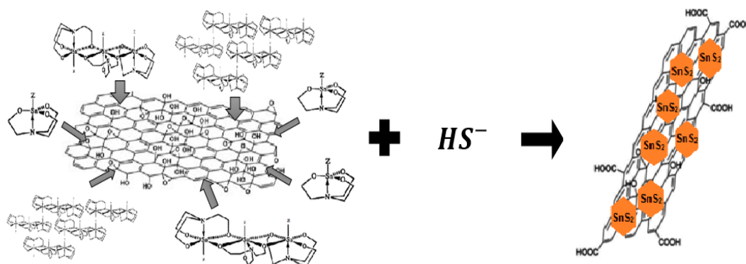
Figura N° 9. Esquema de formación del material compuesto \text{SnS}_2/\text{GO}
