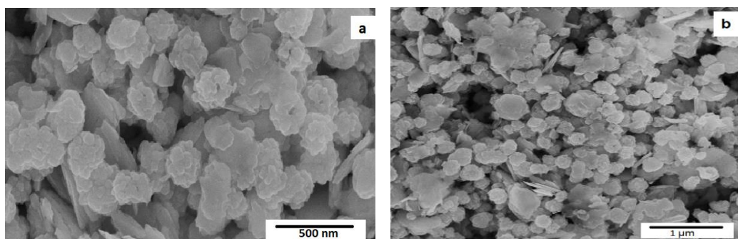
Figura N° 7. Micrografías SEM. \text{SnS}_2 -6H (a) Cristal (b) Aglomerado
