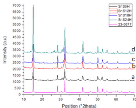
Figura N° 6. Espectros de difracción de rayos X. a) \text{SnS}_2 -6H. b) \text{SnS}_2 -12H. c) \text{SnS}_2 -18H d) \text{SnS}_2 -24H
