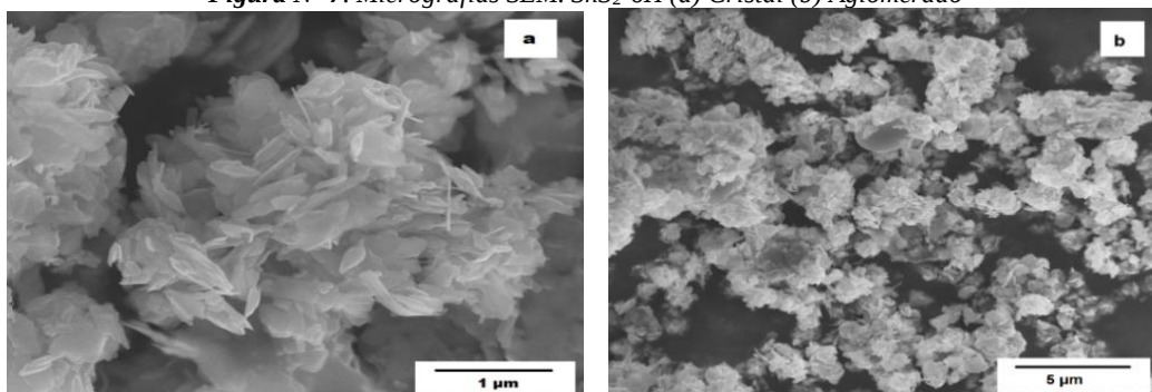
Figura N° 8. Micrografías SEM. \text{SnS}_2 -24H (a) Cristal (b) Aglomerado
