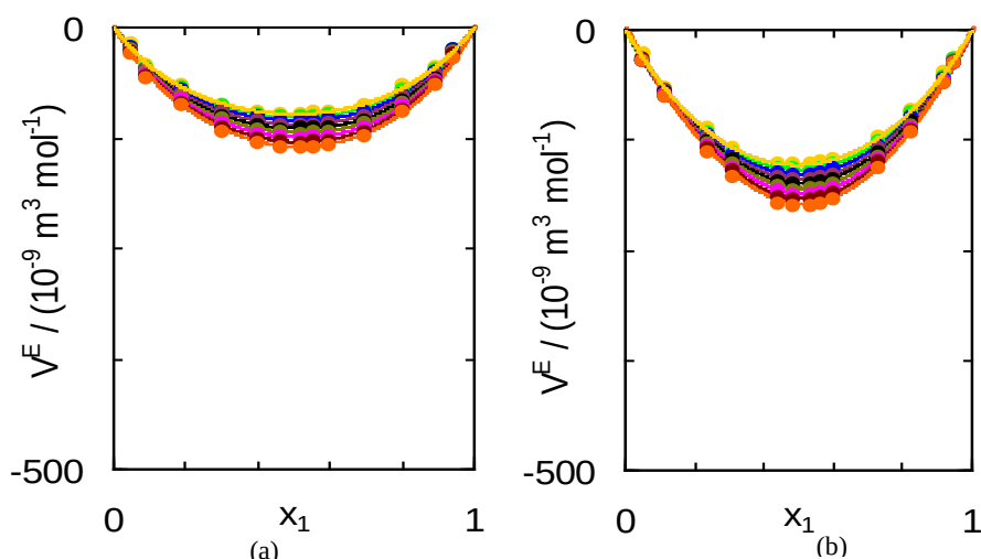
Figura 1. Volúmenes molares de exceso, V^E , de los sistemas x propanonitrilo + (1-x) propanoato de metilo(a), x propanonitrilo + (1-x) propanoato de etilo (b) a las temperaturas de: ● 278.15 K, ● 283.15 K, ● 288.15 K, ● 293.15 K, ● 298.15 K, ● 303.15 K, ● 308.15 K, ● 313.15 K, ● 318.15 K.
