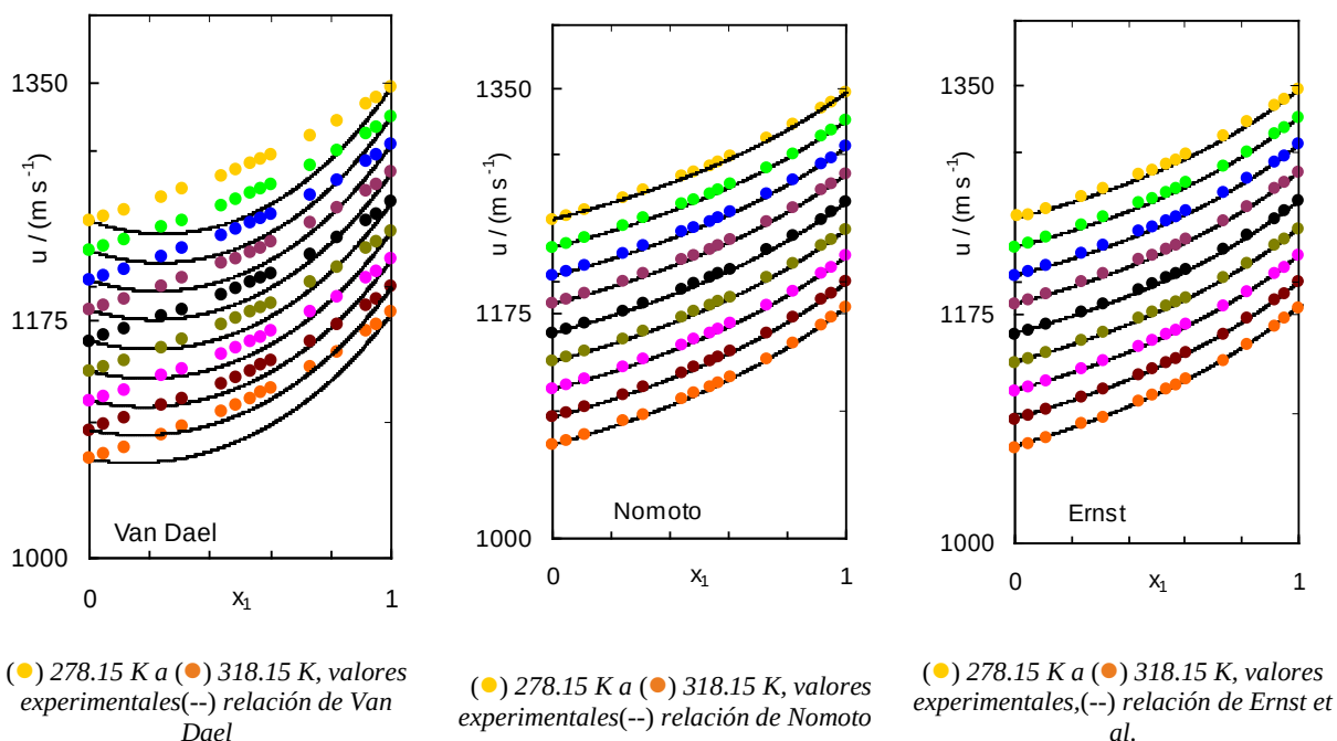
Figura 3. Comparación entre valores teóricos y experimentales de velocidades del sonido, u , del sistema x propanonitrilo + (1-x) propanoato de metilo a las temperaturas de: ● 278.15 K, ● 283.15 K, ● 288.15 K, ● 293.15 K, ● 298.15 K, ● 303.15 K, ● 308.15 K, ● 313.15 K, ● 318.15 K.
