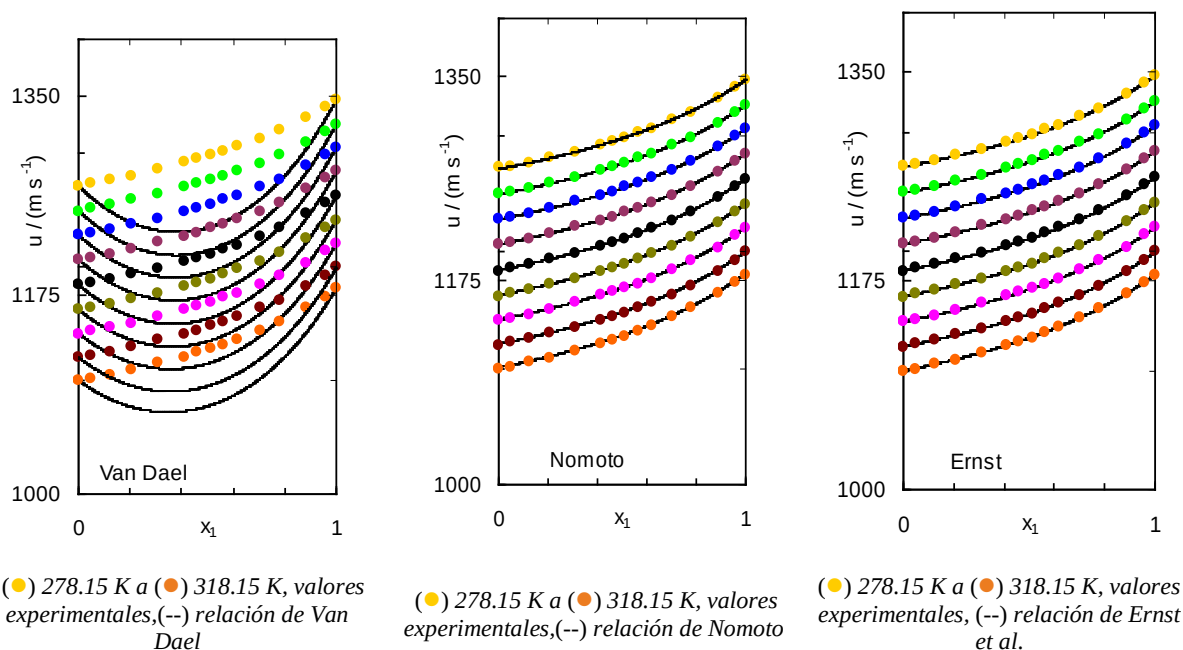
Figura 4. Comparación entre valores teóricos y experimentales de velocidades del sonido, u , del sistema x propanonitrilo + (1-x) propanoato de etilo a las temperaturas de: ● 278.15 K, ● 283.15 K, ● 288.15 K, ● 293.15 K, ● 298.15 K, ● 303.15 K, ● 308.15 K, ● 313.15 K, ● 318.15 K.
