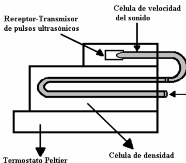
Figura 6. Células de medida de la densidad y de la velocidad de sonido en el DSA-48.
