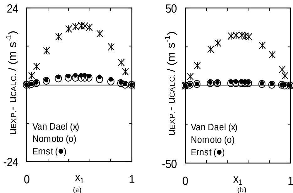
Figura 5. Desviaciones de la velocidad del sonido, valores experimentales respecto de calculados con los modelos de predicción, mediante la relación de mezcla ideal de Van Dael (x), la relación empírica de Nomoto (o), y el modelo de velocidad media de Ernst u_{EXP} - u_{CALC.} , para cada fracción molar, y a 298.15 K de los sistemas x propanonitrilo + (1-x) propanoato de metilo(a) y x propanonitrilo + (1-x) propanoato de etilo (b).
