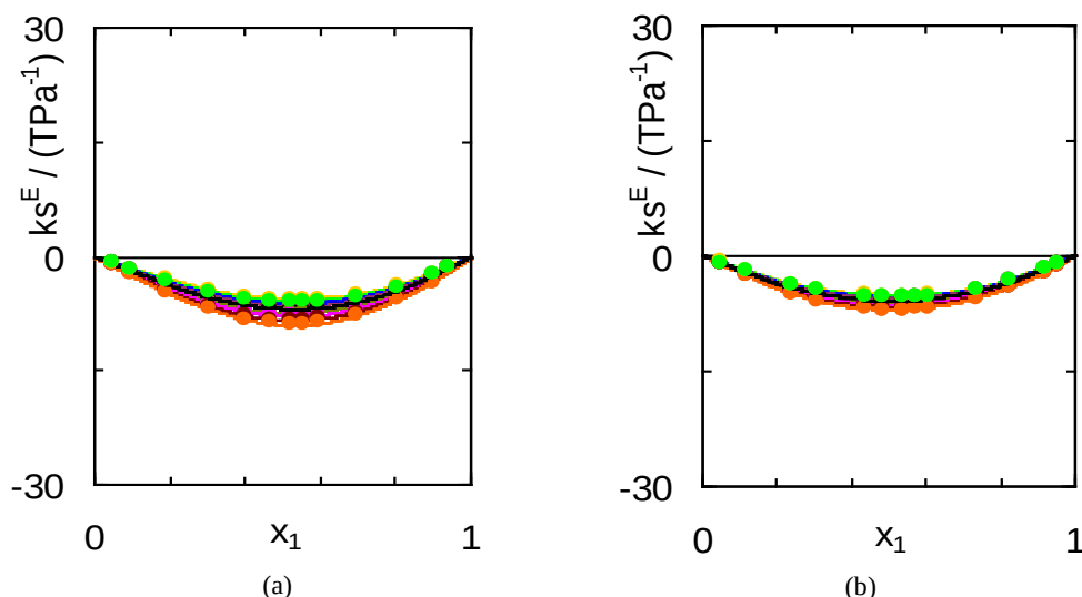
Figura 2. Compresibilidades isoentrópicas de exceso, K_S^E de los sistemas x propanonitrilo + (1-x) propanoato de metilo (a), x propanonitrilo + (1-x) propanoato de etilo (b) ● 278.15 K, ● 283.15 K, ● 288.15 K, ● 293.15 K, ● 298.15 K, ● 303.15 K, ● 308.15 K, ● 313.15 K, ● 318.15 K.
