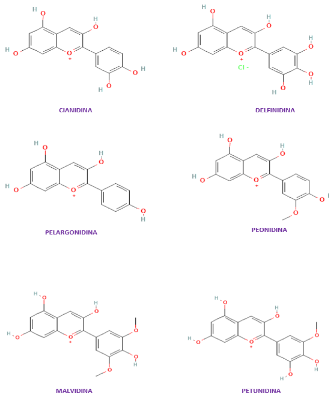
Figura 2. Antocianidinas: Estructura de las antocianidinas más comunes en plantas con el respectivo color que manifiestan [4].
