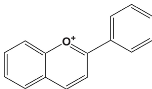
Figura 1. Antocianina: Estructura del ion flavilio [2].
