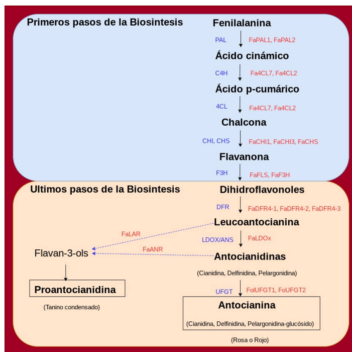
Figura 3. Biosíntesis de Antocianinas: Etapas temprana y tardía de la vía biosintética [8].
