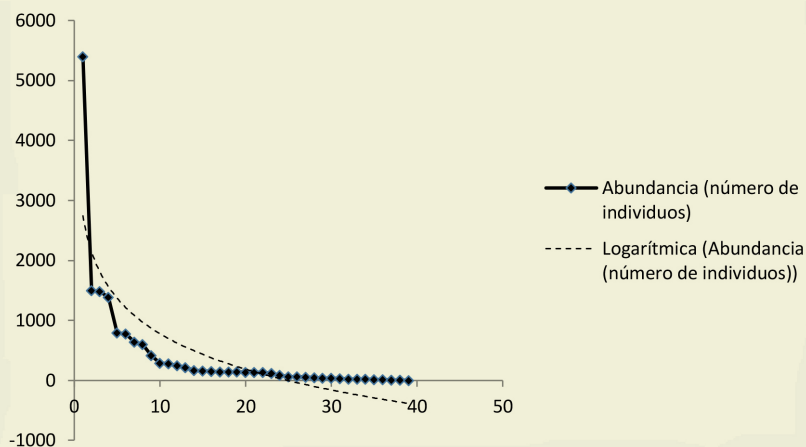
Figura 2. Curva de dominancia-diversidad para las especies del ensamble
