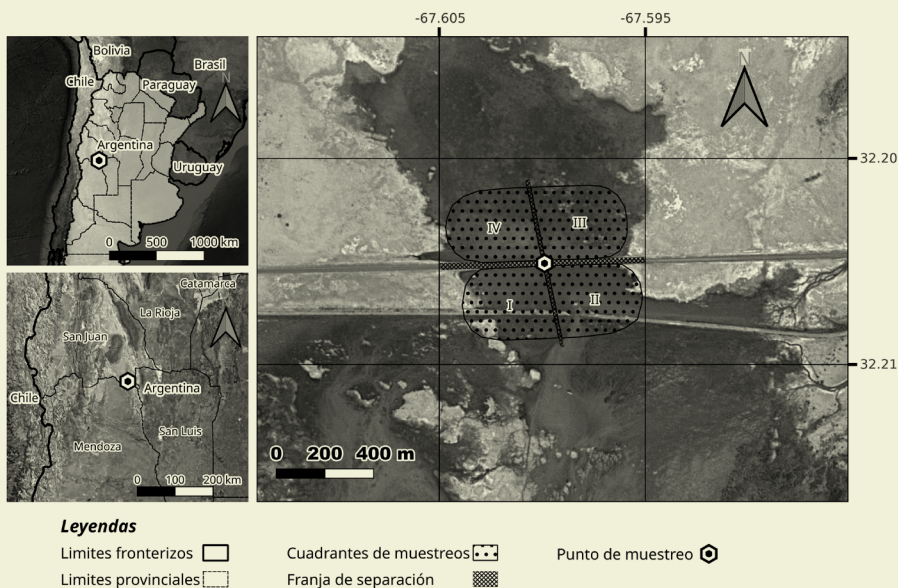
Figura 1. Mapa de localización del área de estudio y cuadrantes de muestreo Figure 1. Location map of the study area and sampling quadrants
