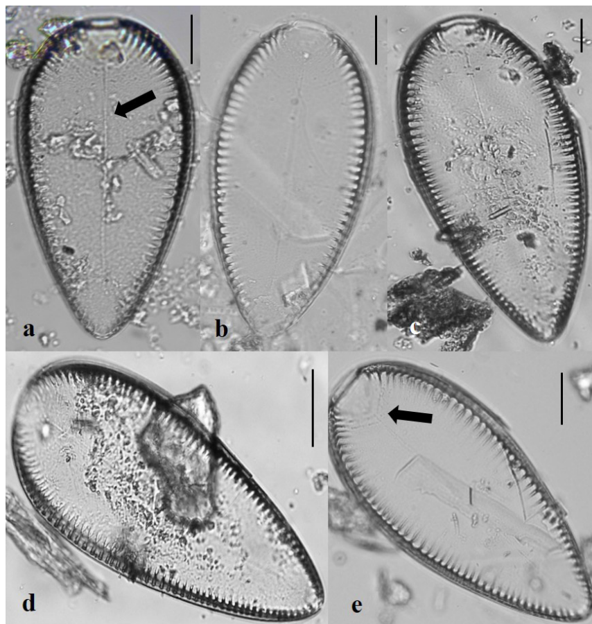
Figura 3. Iconella guatemalensis . Microscopio de luz (100x). Escala de la barra 20 \mu\text{m} . a-e. Vista valvar. a. La flecha indica la línea axial. e. La flecha indica la región cóncava en el polo anterior con la terminación proximal del rafe.
