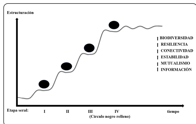
Figura 2. Interpretación de las etapas sucesionales de un matorral xerófilo con tendencia a formar un mezquital mediante cambios graduales. Dominancia de plantas en las etapas serales: I herbáceas anuales y perennes, II arbustos rastreros (< 50 cm), III arbustos medianos (<1.5 m), IV árboles (>2 m). Esquema modificado de Godron (1984).
