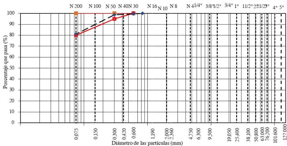
Fig. 6 Curva granulométrica de la ceniza de cáscara de papa (MTC E204/ASTM C136).
