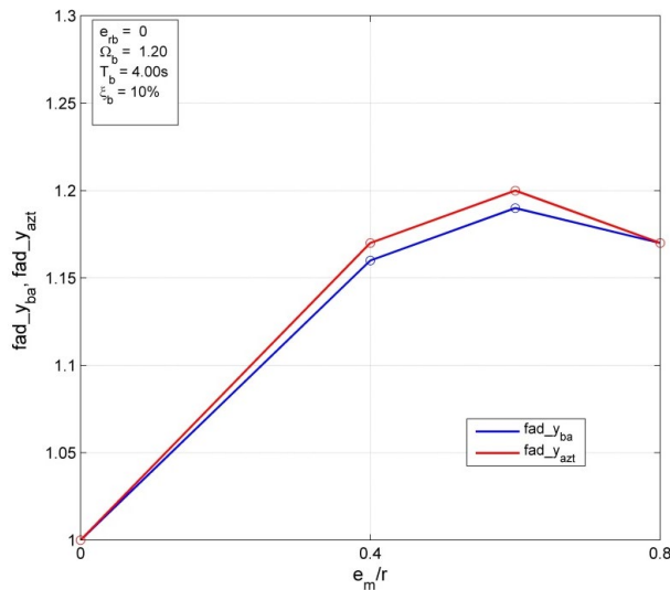
Fig. 4. Efecto de la e_m en el fad_{y_{azt}} y fad_{y_{ba}} para edificios aislados con parámetros e_{rb}/r = 0 , \Omega_b = 1.20 , T_b = 4.0 s y \xi_b = 10\% .
