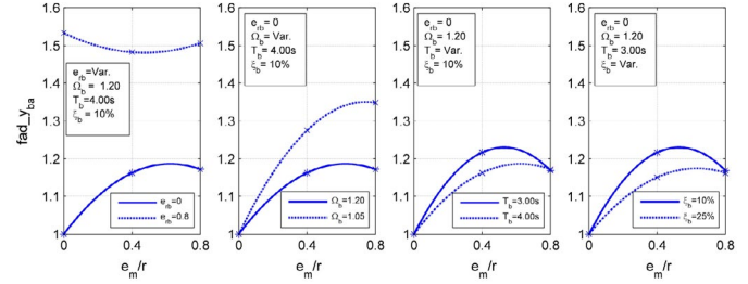
Fig. 5. Efecto de los parámetros e_{rb} , \Omega_b , T_b y \xi_b en fad_{y_{ba}} vs. e_m/r .
