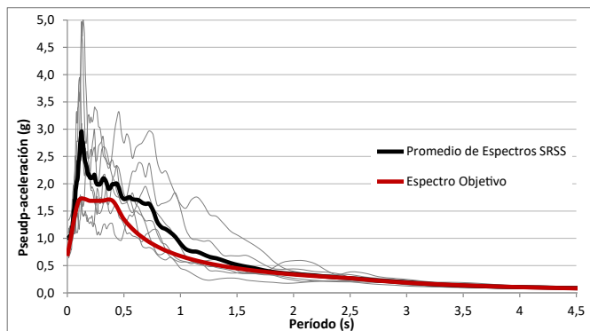
Fig. 3. Escalamiento en amplitud de los siete pares de registros sísmicos respecto al espectro de diseño de la norma peruana E.031
