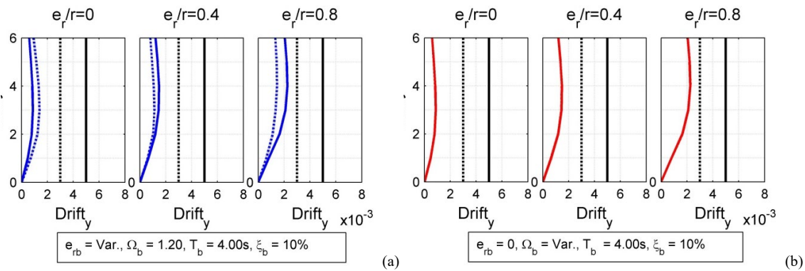
Fig. 13. Efecto de los parámetros e_{rb} , \Omega_b , T_b y \xi_b en derivas, para edificios aislados con e_m : a) Efecto de e_{rb} ,
