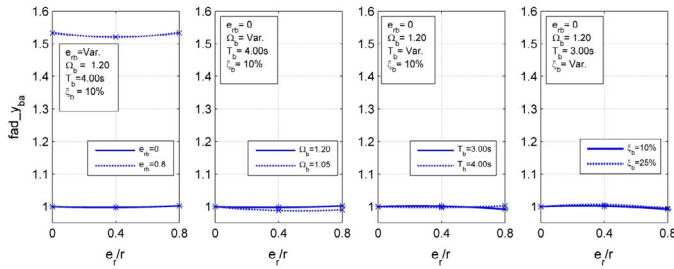
Fig. 7. Efecto de los parámetros e_{rb} , \Omega_b , T_b y \zeta_b en fad_{y_{ba}} vs. e_r/r .
