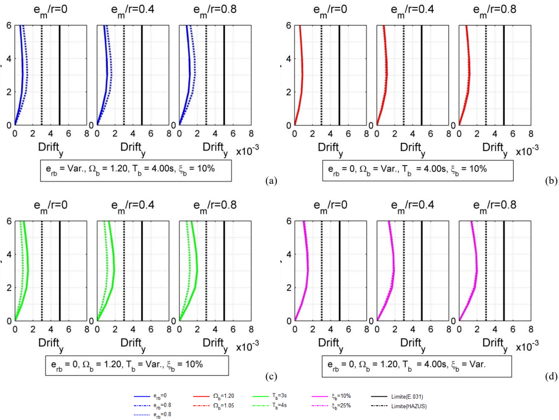
Fig. 13. Efecto de los parámetros e_{rb} , \Omega_b , T_b y \xi_b en derivas, para edificios aislados con e_m : a) Efecto de e_{rb} ,
