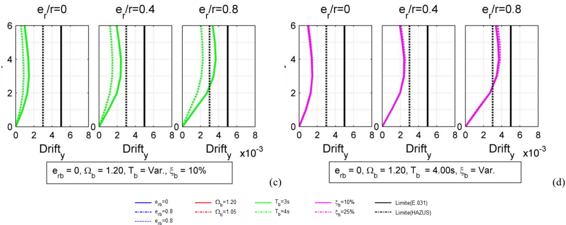
Fig. 14. Efecto de parámetros e_{rb} , \Omega_b , T_b y \xi_b en derivas, para edificios aislados con e_r : a) Efecto de e_{rb} , b) Efecto de \Omega_b , c) Efecto de T_b y d) Efecto de \xi_b .
