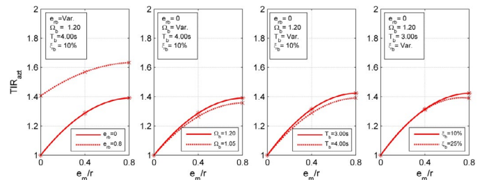
Fig. 10. Efecto de los parámetros e_{rb} , \Omega_b , T_b y \zeta_b en TIR_{azt} vs. e_m/r .
