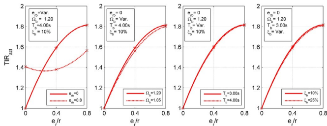
Fig. 12. Efecto de los parámetros e_{rb} , \Omega_b , T_b y \xi_b en TIR_{azt} vs. e_r/r .
