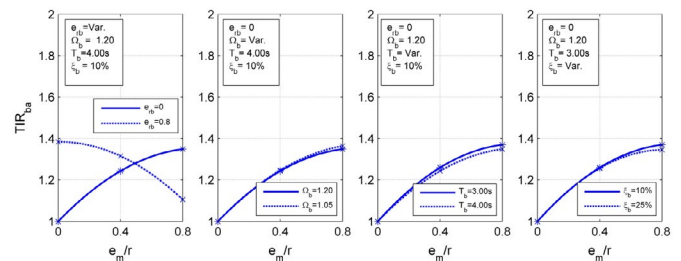
Fig. 9. Efecto de los parámetros e_{rb} , \Omega_b , T_b y \zeta_b en TIR_{ba} vs. e_m/r .
