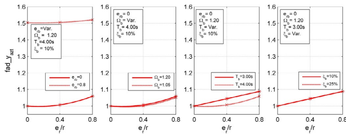
Fig. 8. Efecto de los parámetros e_{rb} , \Omega_b , T_b y \zeta_b en fad_{y_{azt}} vs. e_r/r .
