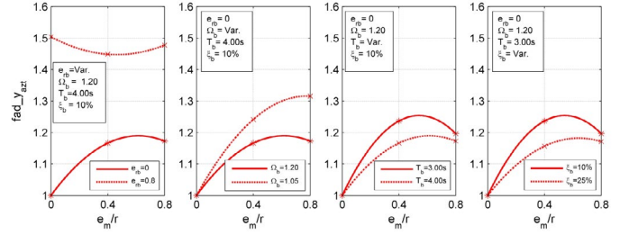
Fig. 6. Efecto de los parámetros e_{rb} , \Omega_b , T_b y \xi_b en fad_{y_{azt}} vs. e_m/r .
