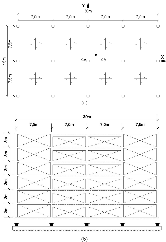
Fig. 2. Configuración de modelos estructurales: a) Planta estructural típica y b) Elevación típica.
