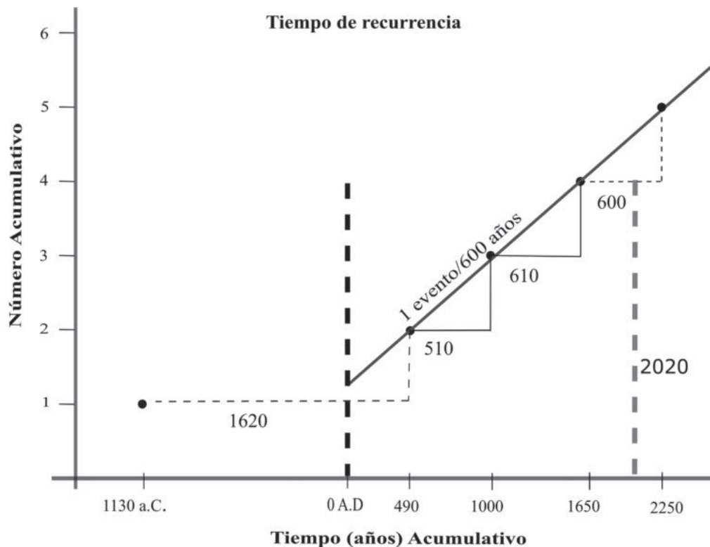
Fig. 11: Estimación de la recurrencia. La línea recta inclinada es la de mejor ajuste. La línea punteada en negro marca el año cero de nuestra era. El último punto de la recta representa la proyección de una erupción en el futuro, la cual correspondería al año 2250. La línea punteada gris representa el año 2020.
