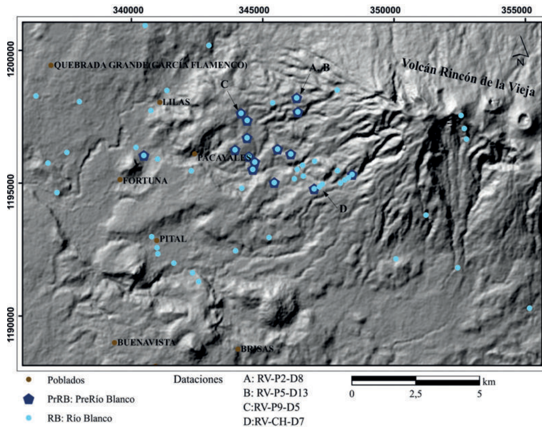
Fig. 5: Ubicación cortes artificiales donde se observaron y midieron los depósitos de RB y PrRB.
