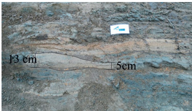
Fig. 3: Capas de cenizas lentiformes interpretadas como corrientes de densidad piroclástica diluida del 3650 a. C., a los 4 m desde la superficie se encuentran estas capas de ceniza con acuñamientos (1197694N/346336E).
