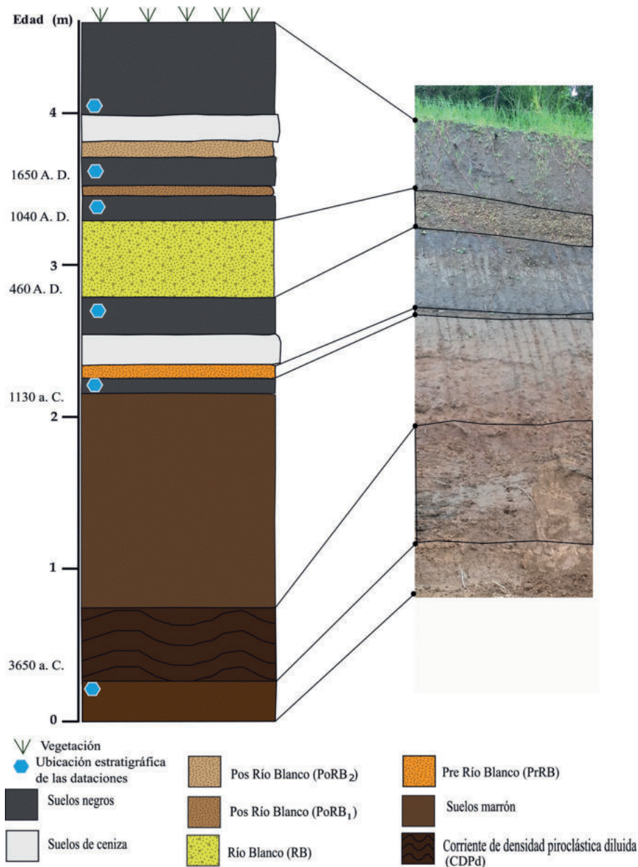
Fig. 2: Columna estratigráfica: representación de los distintos niveles estudiados en campo con un afloramiento (1197694N/346336E). Las edades de las dataciones se presentan en el Cuadro 2.
