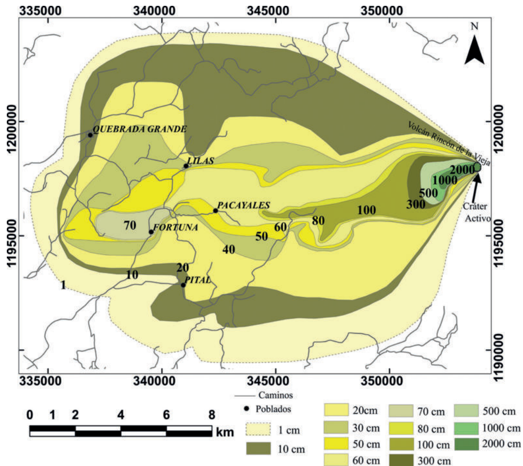
Fig. 7: Isopacas de la pliniana RB, se observa cómo se dan dos máximos, uno cercano al cráter y otro al WSW en la parte distal, cerca de Fortuna. Elaborado a partir de la integración de datos de campo de Kempter (1997), Barahona et al. (2001) y el presente trabajo.
