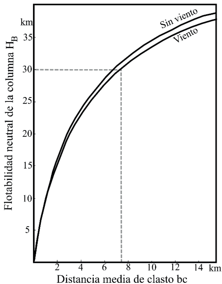
Fig. 8: Diagrama de Pyle (1989), modificado para estimar la altura de la columna eruptiva de Río Blanco.
