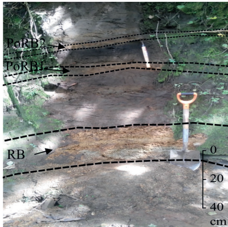
Fig. 9: Detalle de los eventos posteriores a Río Blanco, PoRB1 y PoRB2, intercalados por cenizas grises (1195012N/347957E).
