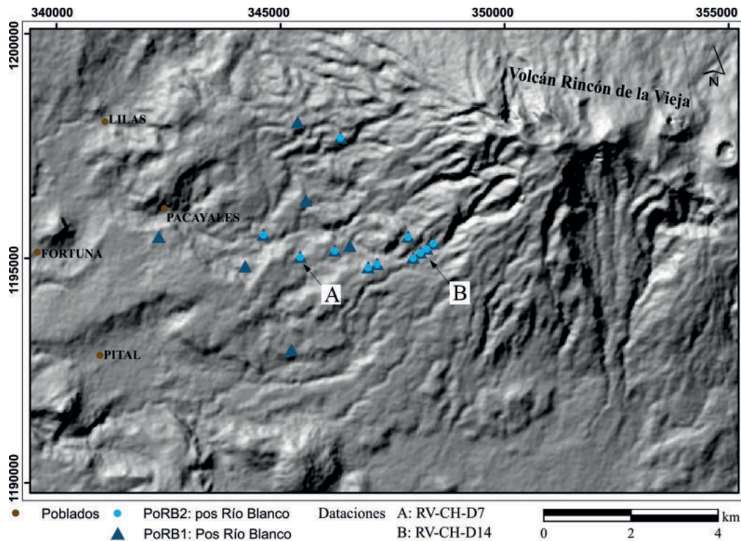
Fig. 10: Ubicación de los sitios donde se observa estas nuevas capas propuestas y los puntos donde se tomaron las muestras para las dataciones.
