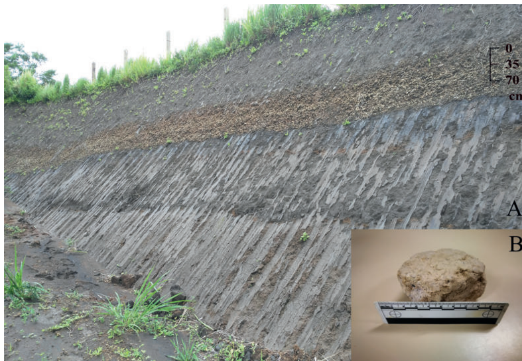
Fig. 6: A) Depósito de la capa pliniana RB (1197694N/346336E). B) Pómez de 8 x 6 cm.
