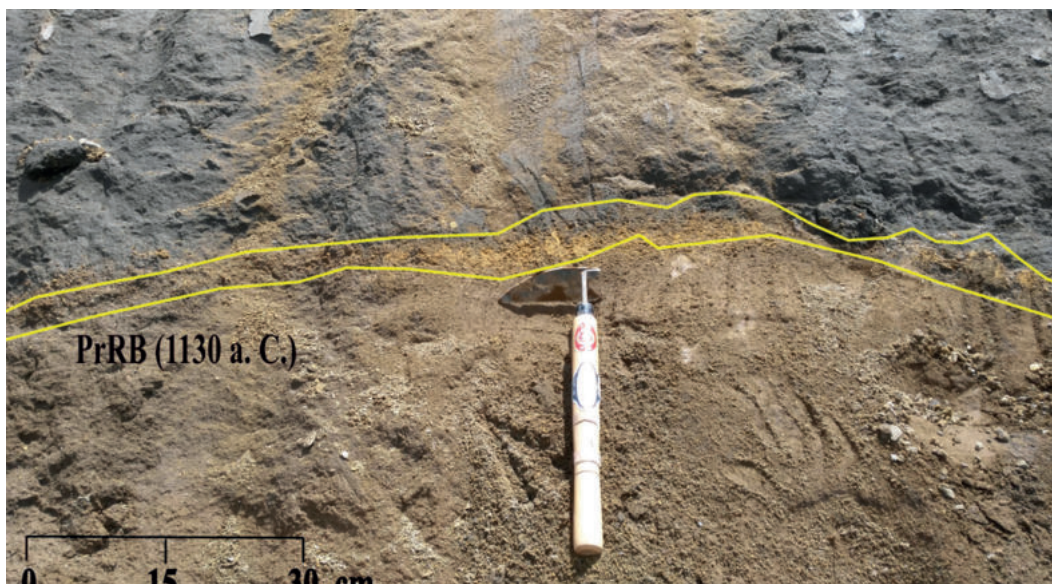
Fig. 4: Capa PrRB resaltada en amarillo, cuya edad fue determinada en 1130 a. C. (1196288N/345567E).
