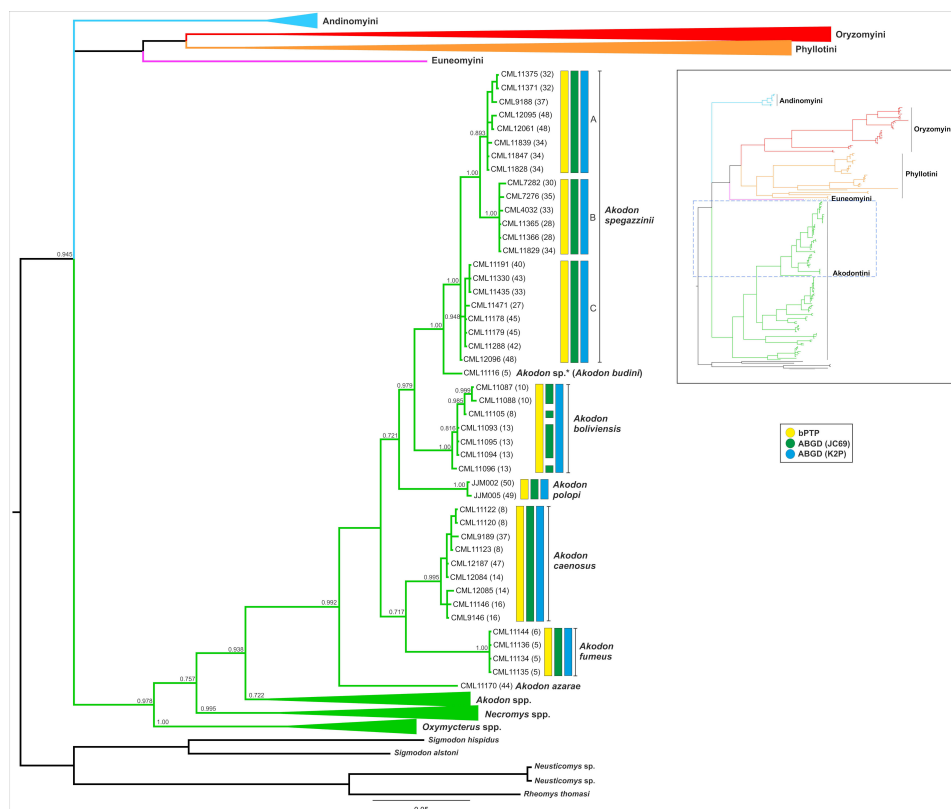
Fig. 4. Árbol de consenso de mayoría obtenido mediante inferencia bayesiana: relaciones filogenéticas para parte de los especímenes representantes de la tribu Akodontini. Para detalles adicionales, véase el Fig. 2. La secuencia CML 11116 ( Akodon sp.) proviene de un ejemplar perteneciente a Akodon budini .
