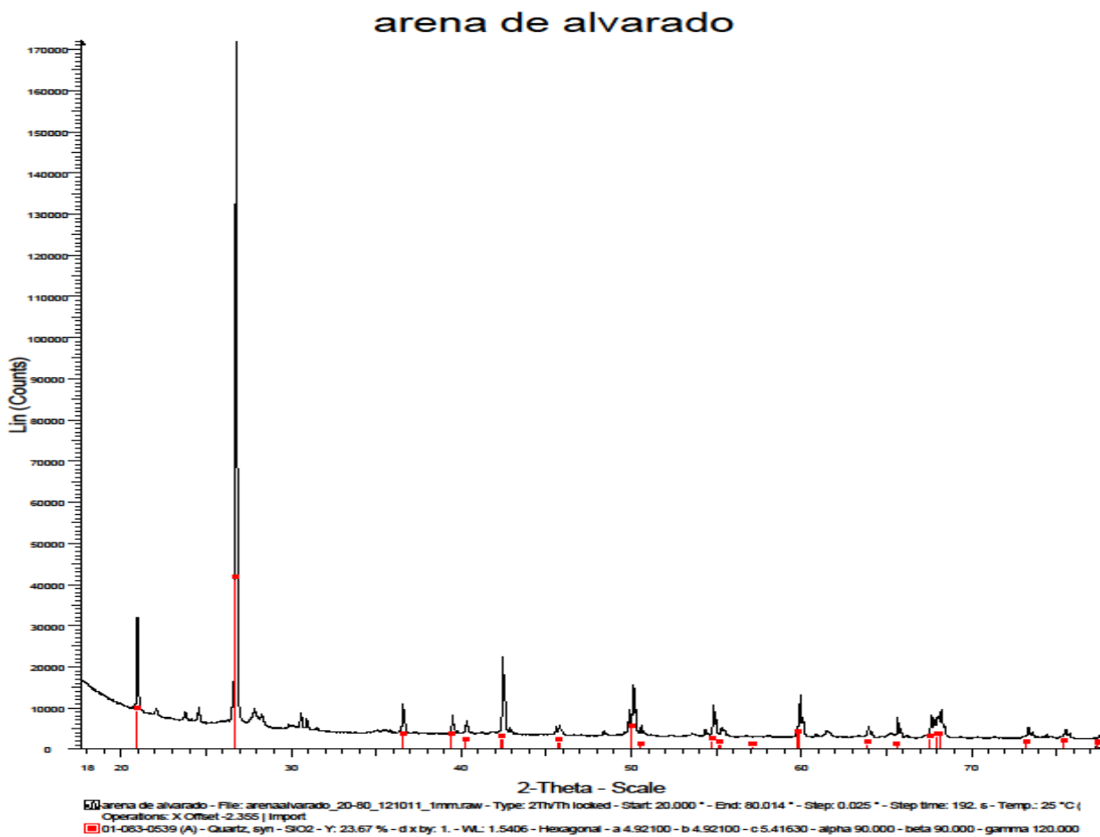
Figura 6. Resultados de la difracción de rayos X.
