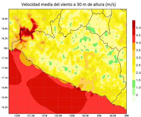
Figura 2. Velocidad media del viento a 30 m de altura
