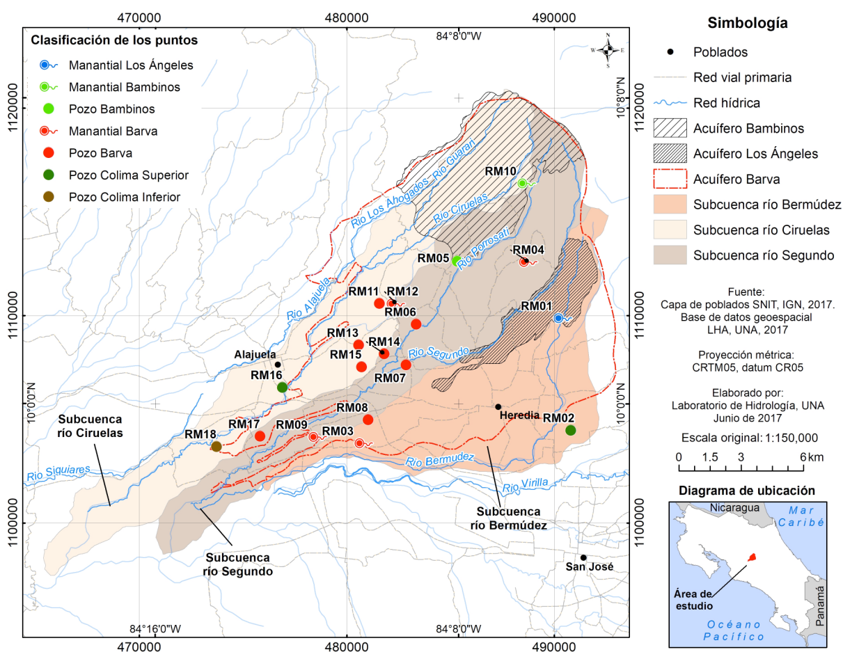
Figura 4. Ubicación de los pozos y manantiales que conforman la red de monitoreo de calidad física y química para aguas subterráneas de los acuíferos Barva y Colima en las subcuencas de los ríos Bermúdez, Ciruelas y Segundo, Costa Rica. Elaboración propia.
