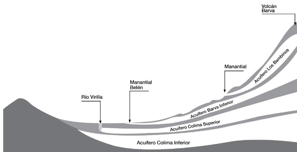
Figura 2. Corte transversal simplificado de los acuíferos en el sector noroeste del Valle Central. Elaboración propia.
