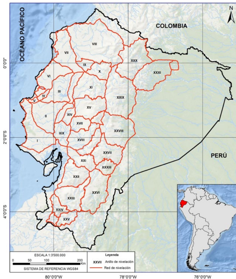
Figura 1. Red de nivelación del Ecuador.
