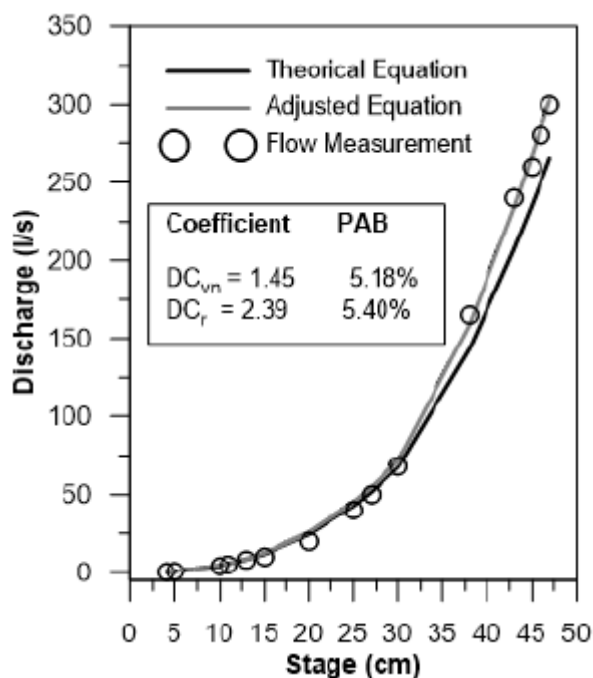
Figura 4. Calibración de la curva de descarga para el vertedero compuesto M4.
