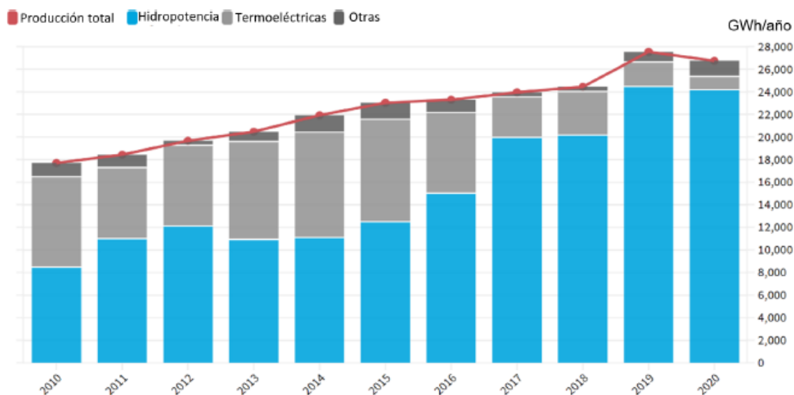
Figura 3. Producción energética Ecuador GWh / año. Fuente: CELEC (2020).
