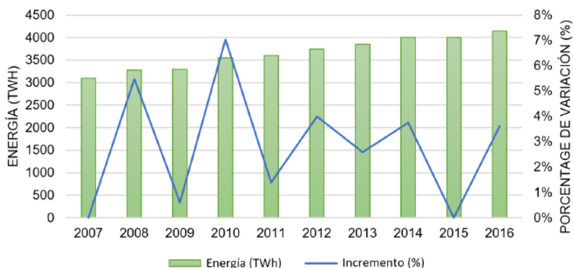
Figura 1. Crecimiento hidroeléctrico mundial TWh período 2007 - 2016. Fuente: International Renewable Energy Agency (2020) y Killingtveit (2018).
