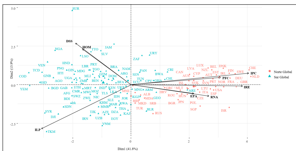
Figura 4. Biplot del plano 1-2 en el análisis PCA según países del norte y sur global.
