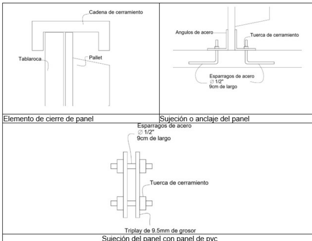
Figura 7. Detalles de conexión y unión entre tarimas y sujeción inferior y superior del módulo.
