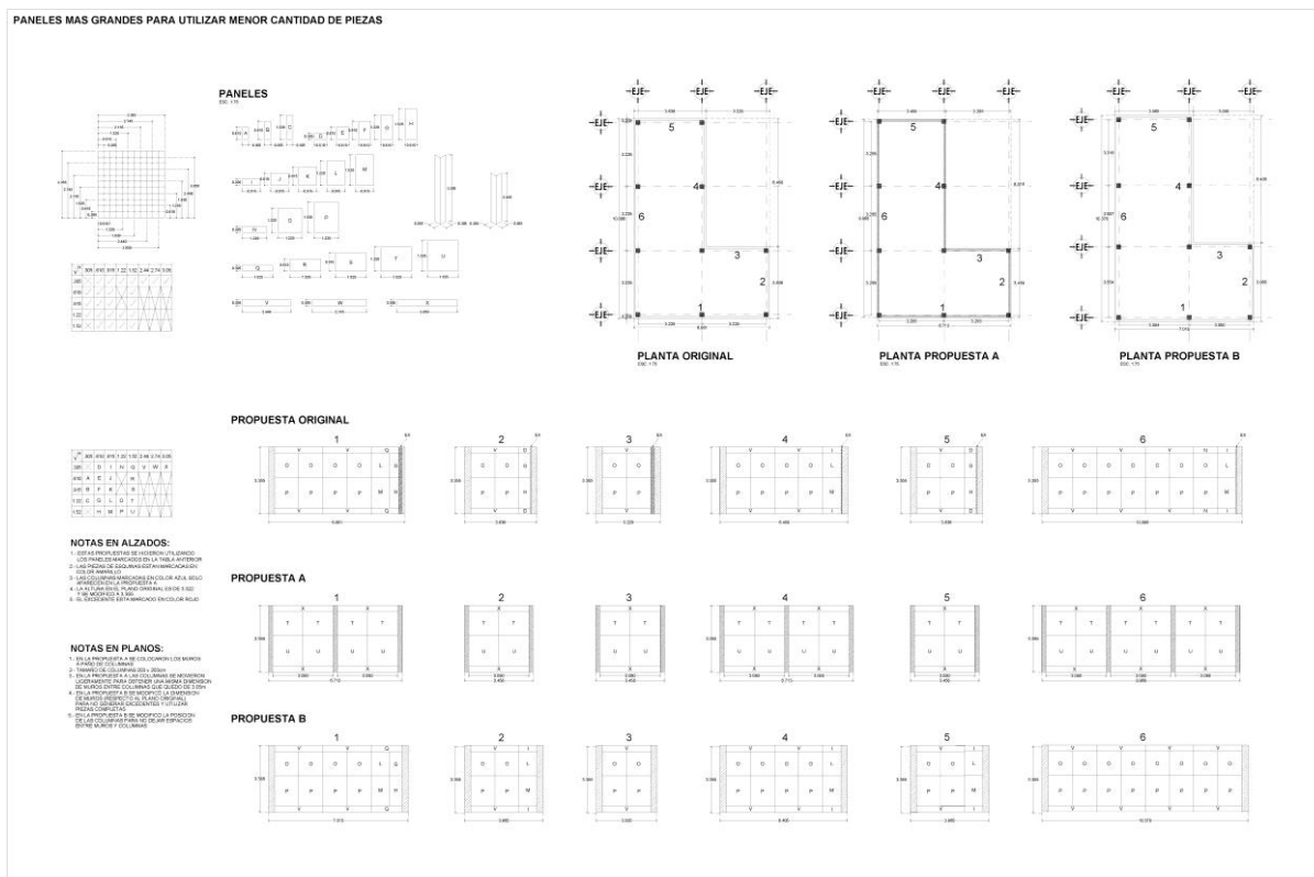
Figura 4. Modulaci3n de objeto de dise1o.
