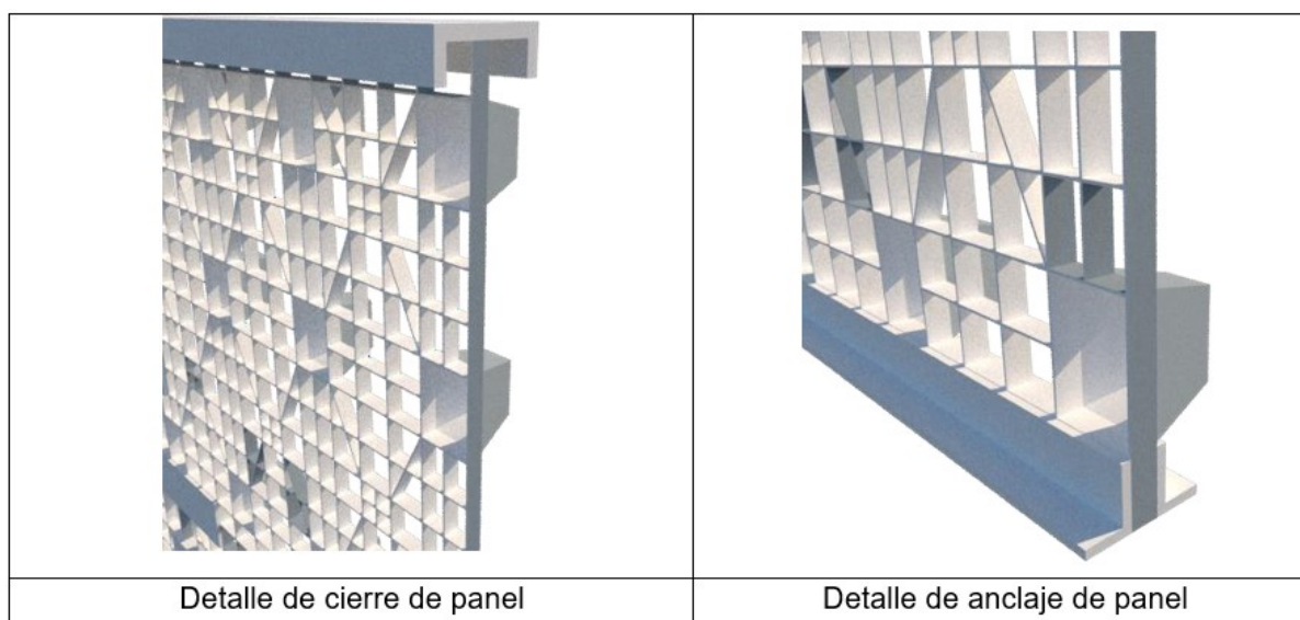
Figura 8. Detalles en isométrico de anclaje a piso y sujeción en cubierta.
