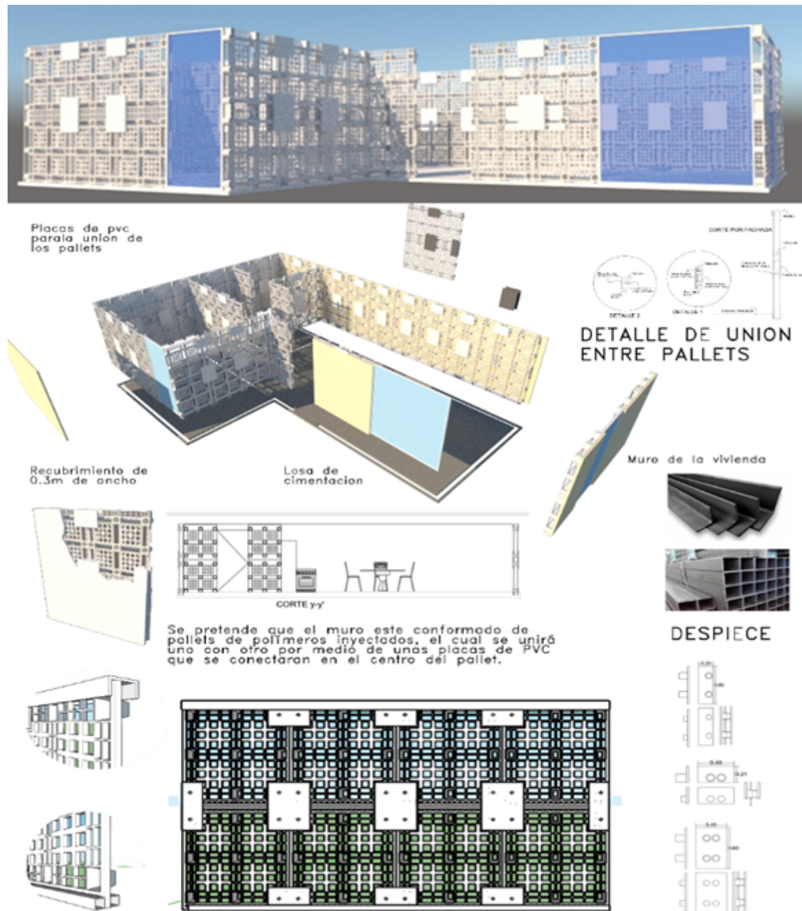
Figura 6. Conexiones de tarimas.
