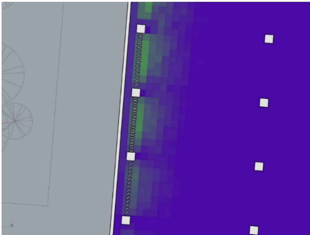
Figura 13 . Radiación con persianas verticales interiores en diferentes ángulos.
