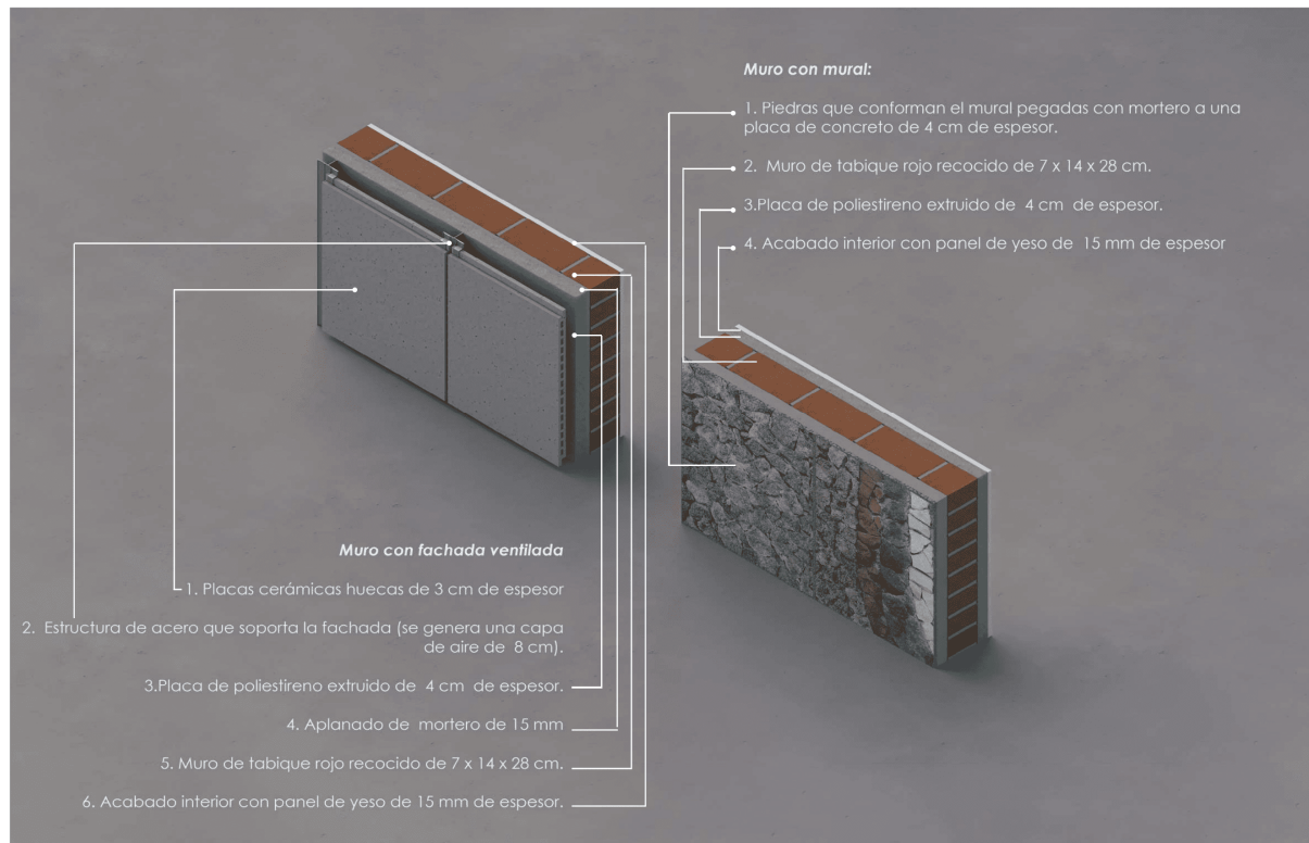
Figura 3. Modelo de propuestas para los distintos tipos de muros en fachada.
