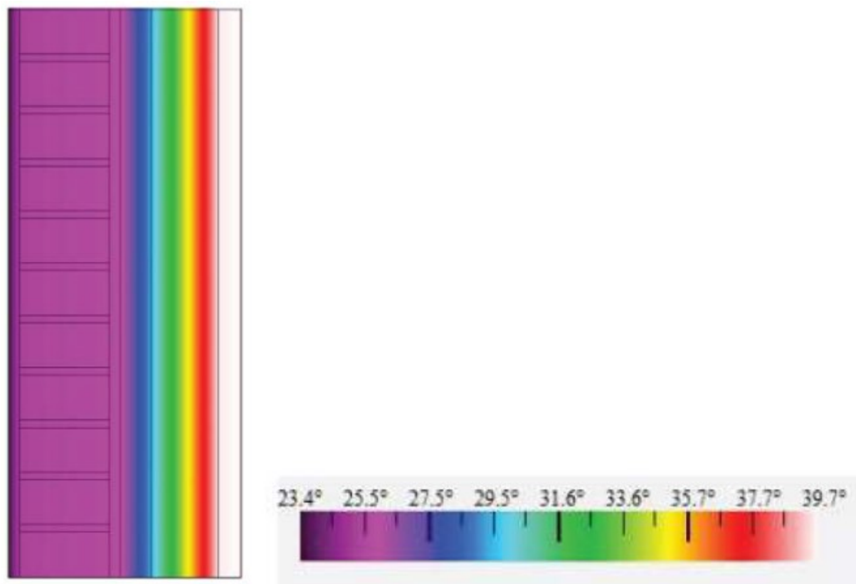
Figura 5. Modelo energético de muro de propuesta. Fuente: Elaboración propia.
