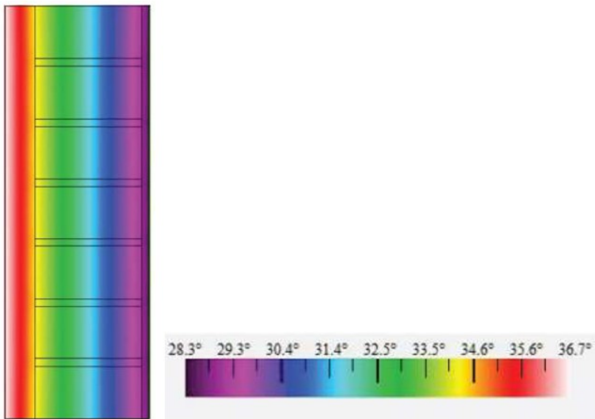
Figura 4. Modelo energético de muro con concreto actual.
