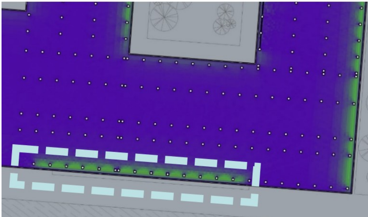
Figura 10 . Energía solar en fachada sur sin elemento de sombreado.
