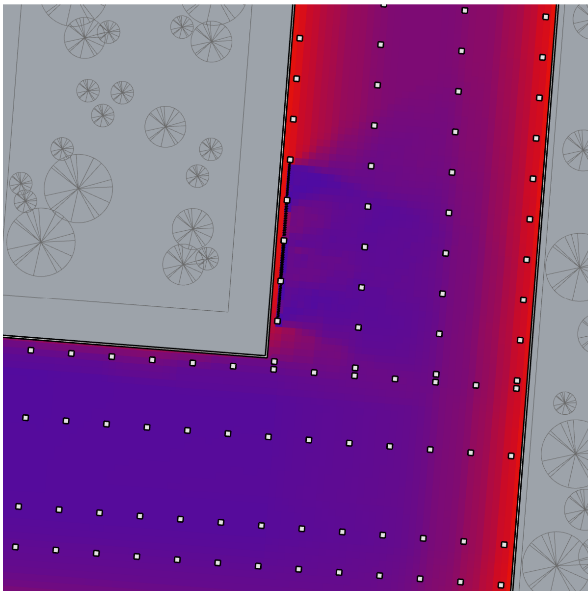
Figura 15 . Gráfica de horas con luz natural con los elementos de sombreado en la fachada oeste.
