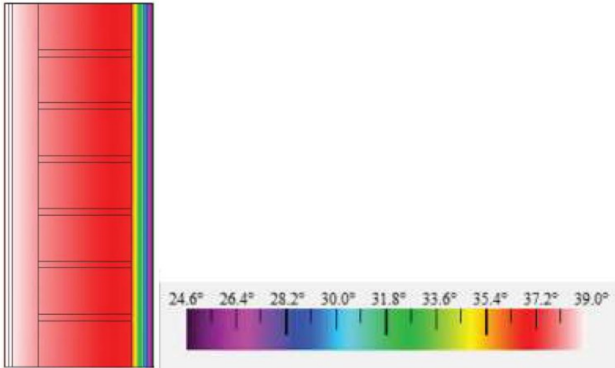
Figura 7. Modelo energético de muro con mural de propuesta. Fuente: Elaboración propia.
