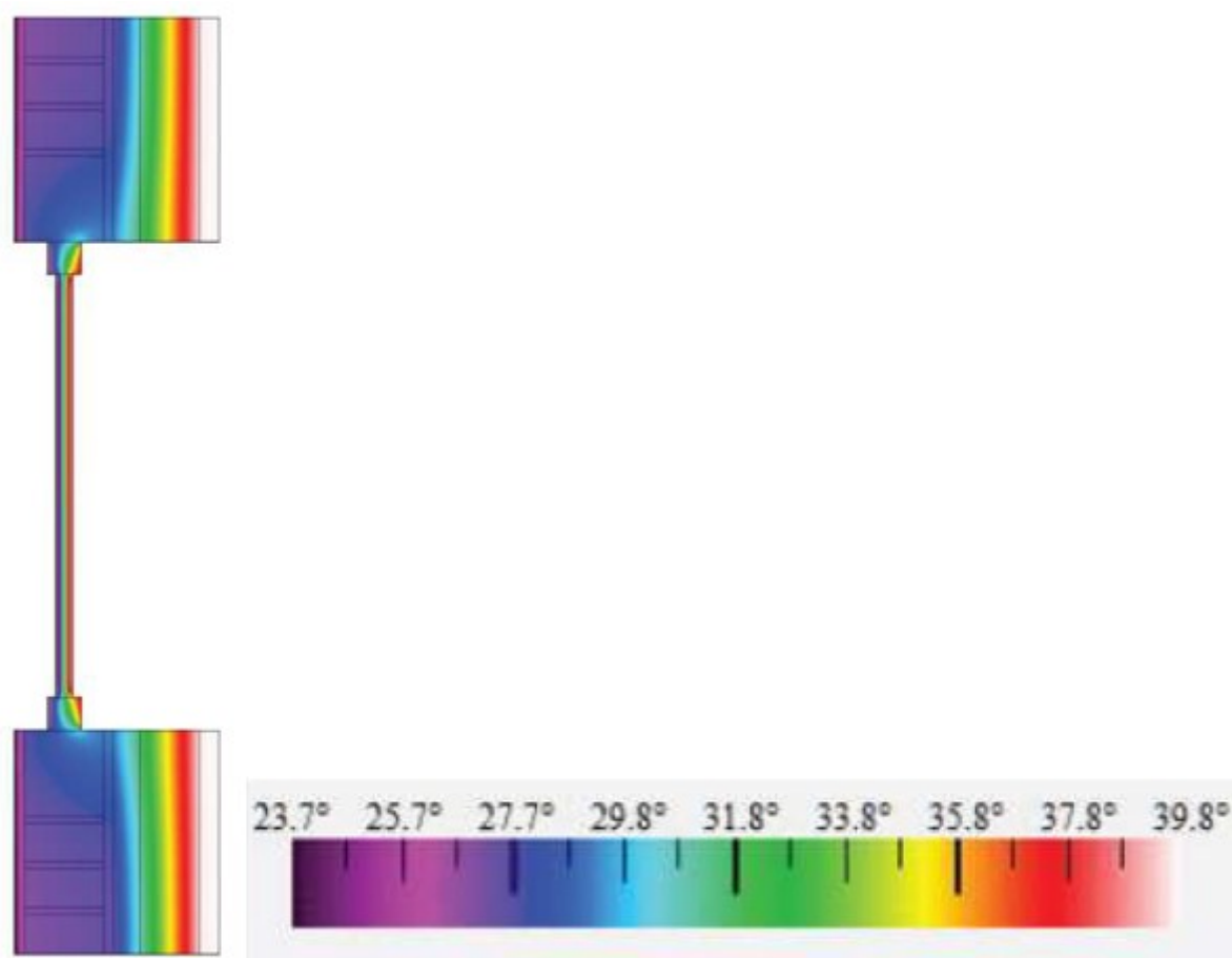
Figura 2. Modelo energético de ventana propuesta.
