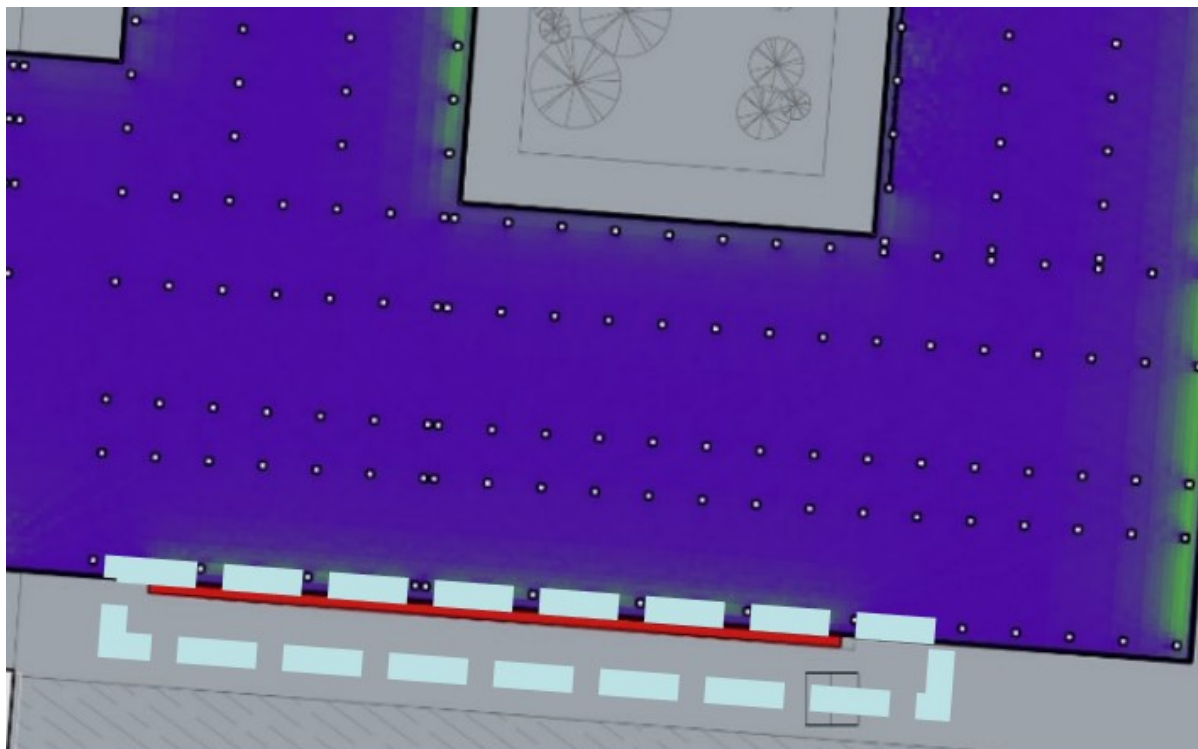
Figura 11 . Energía solar en fachada sur con elemento de sombreado.
