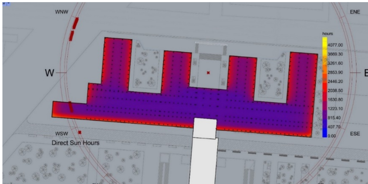
Figura 14 . Gráfica de horas con luz natural sin elementos de sombreado (estado actual). Fuente: Elaboración propia.
