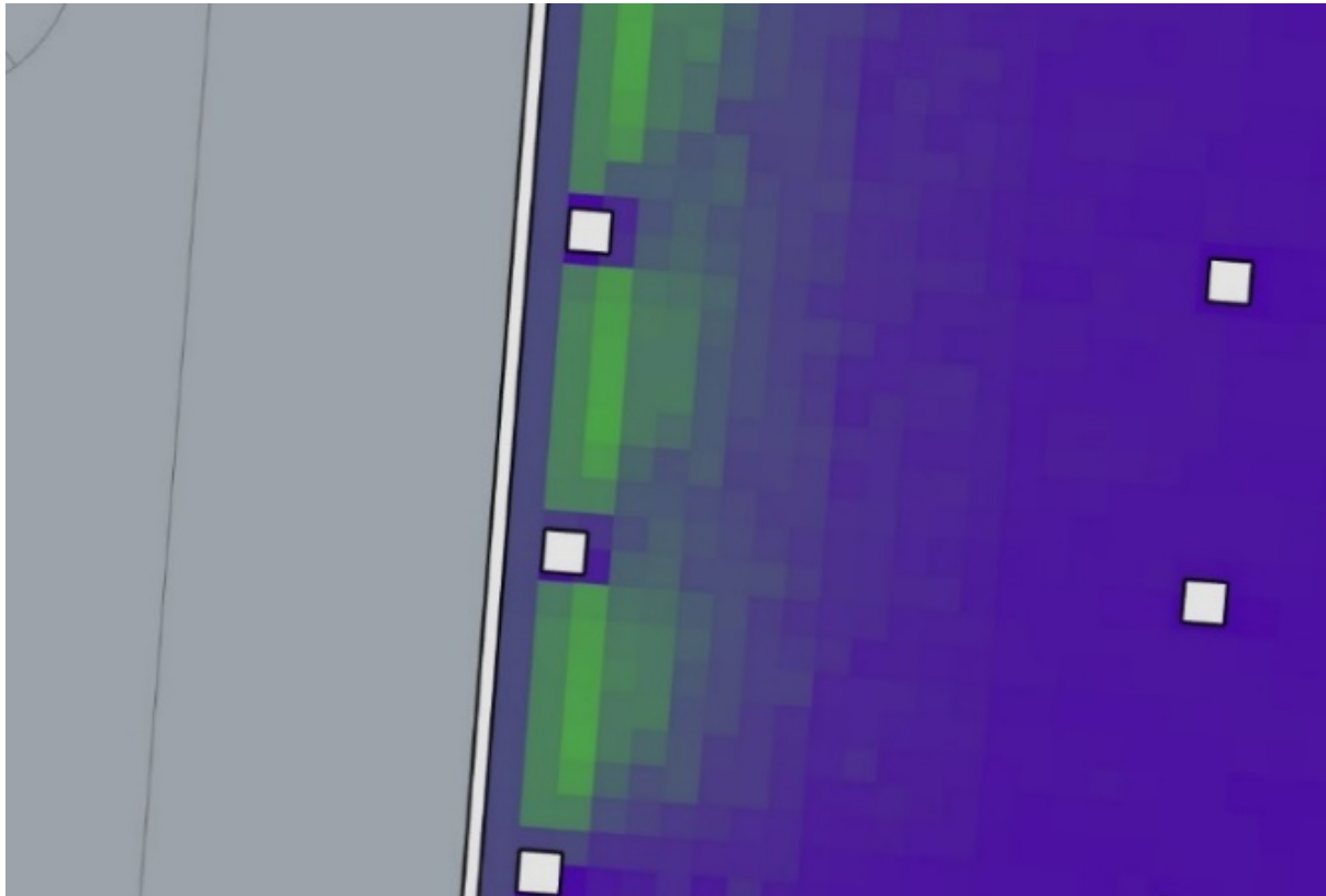
Figura 12 . Estado actual de la radiación solar en losa en fachada oeste sin elementos de sombreado.
