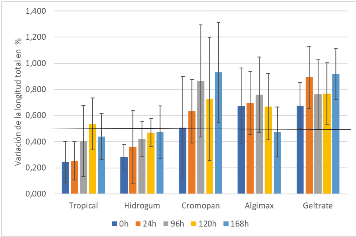
Fig. 5. Variación de la longitud evaluada para cada material respecto al modelo maestro (en %). *Valores positivos representan un aumento en la diferencia de la longitud respecto al modelo maestro. La línea horizontal negra representa el 0.5%, porcentaje máximo de deformación admitido por la mayoría de los estudios.
