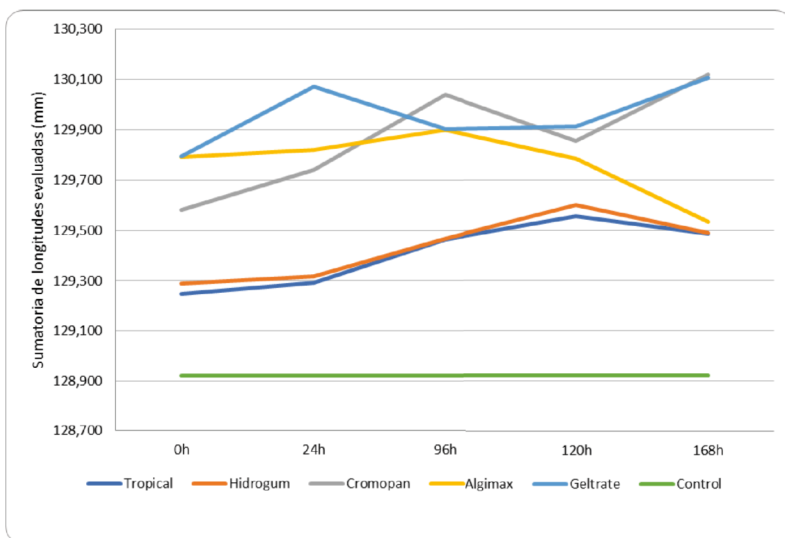
Fig. 4. Sumatoria de las longitudes evaluadas para cada material. Los valores positivos representan un aumento en la diferencia de la longitud respecto al modelo maestro (control).
