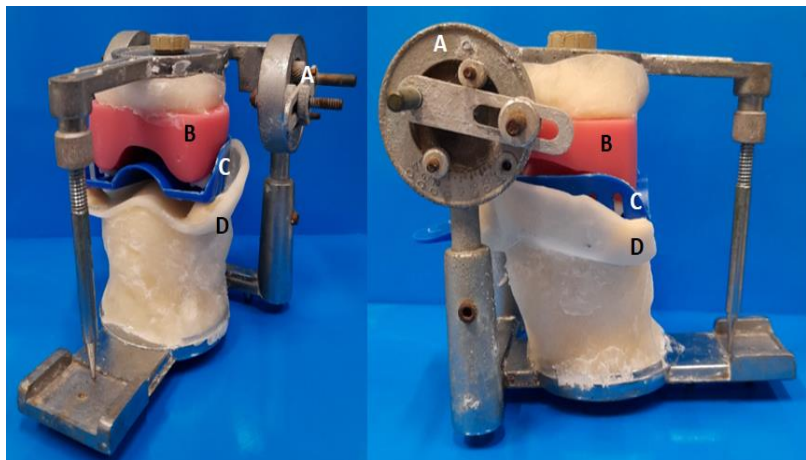
Fig. 1 Representación del dispositivo confeccionado para la estandarización de las impresiones. A) Dispositivo antagonizador de vínculo continuo (articulador). B) Modelo maestro de acrílico fijado a la rama superior del dispositivo. C) Cubeta de stock plástica. D) Base de acrílico confeccionada a medida de la cubeta lo cual permite su estabilización y retiro.
