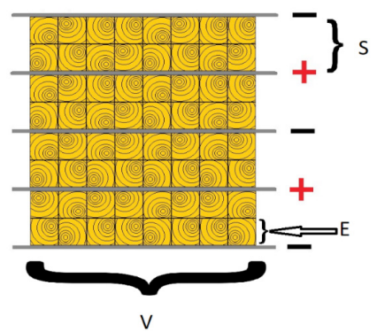
Figura 1. Ejemplo del acomodo de las piezas dentro del equipo, cuya configuración es (E=10cm, S=20 cm y V= 100%).
