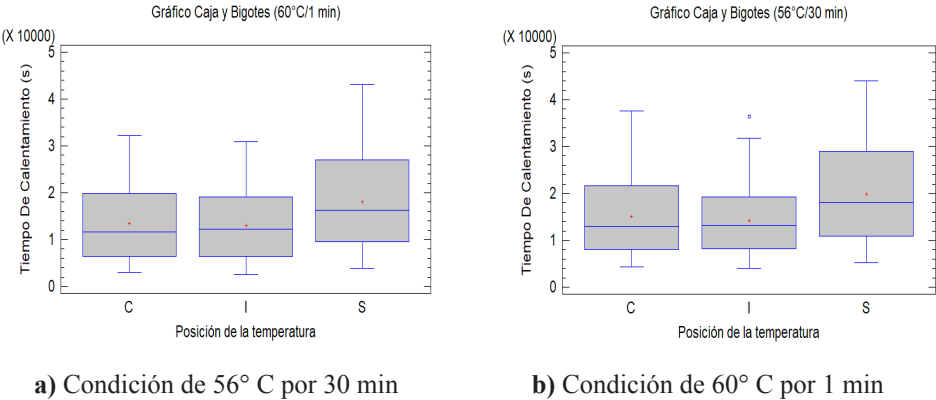
Figura 2. Variación espacial del tiempo de calentamiento por radiofrecuencia. a) Condición 56/30 (°C/min), b) Programa 60/1 (°C/min). Método: 95 porcentaje Duncan C: Central, I: Intermedia, S: Superficie.
