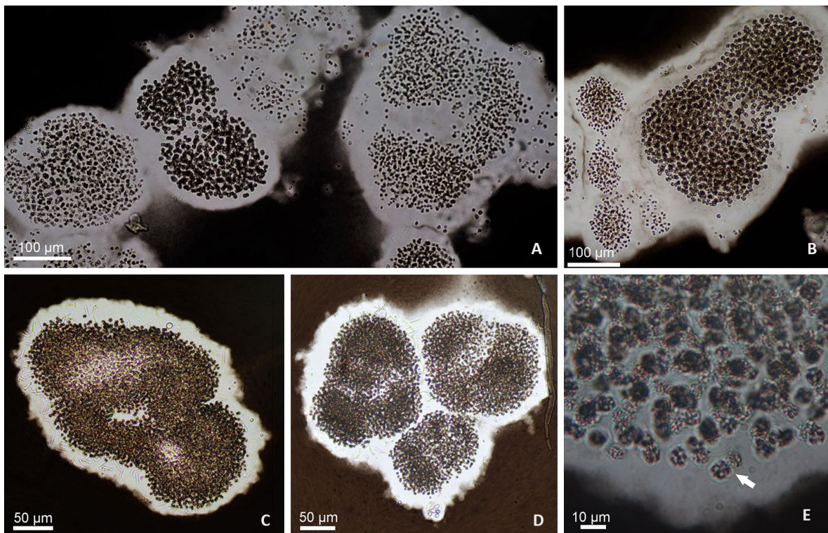
Figura 6. Microcystis aeruginosa .
