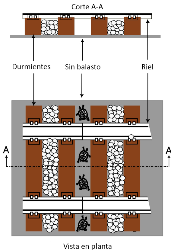
Figura 4. Disposición recomendada de balasto en la vía del tren.
