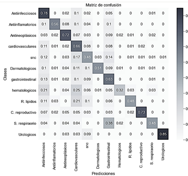
Figura 11. Matriz de confusión con transferencia de aprendizaje (ResNet50) con imágenes 2D más aumentación digital. Fuente: Elaborado por los autores.
