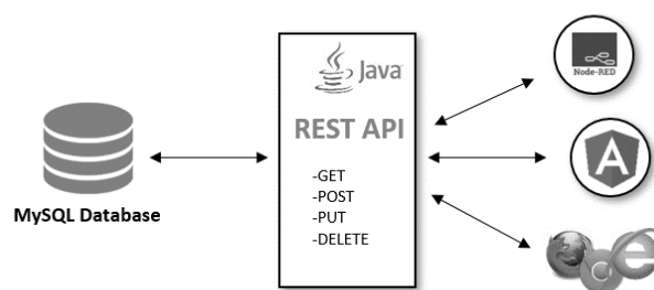
Figura 6. RESTful API. Fuente: Los autores.
