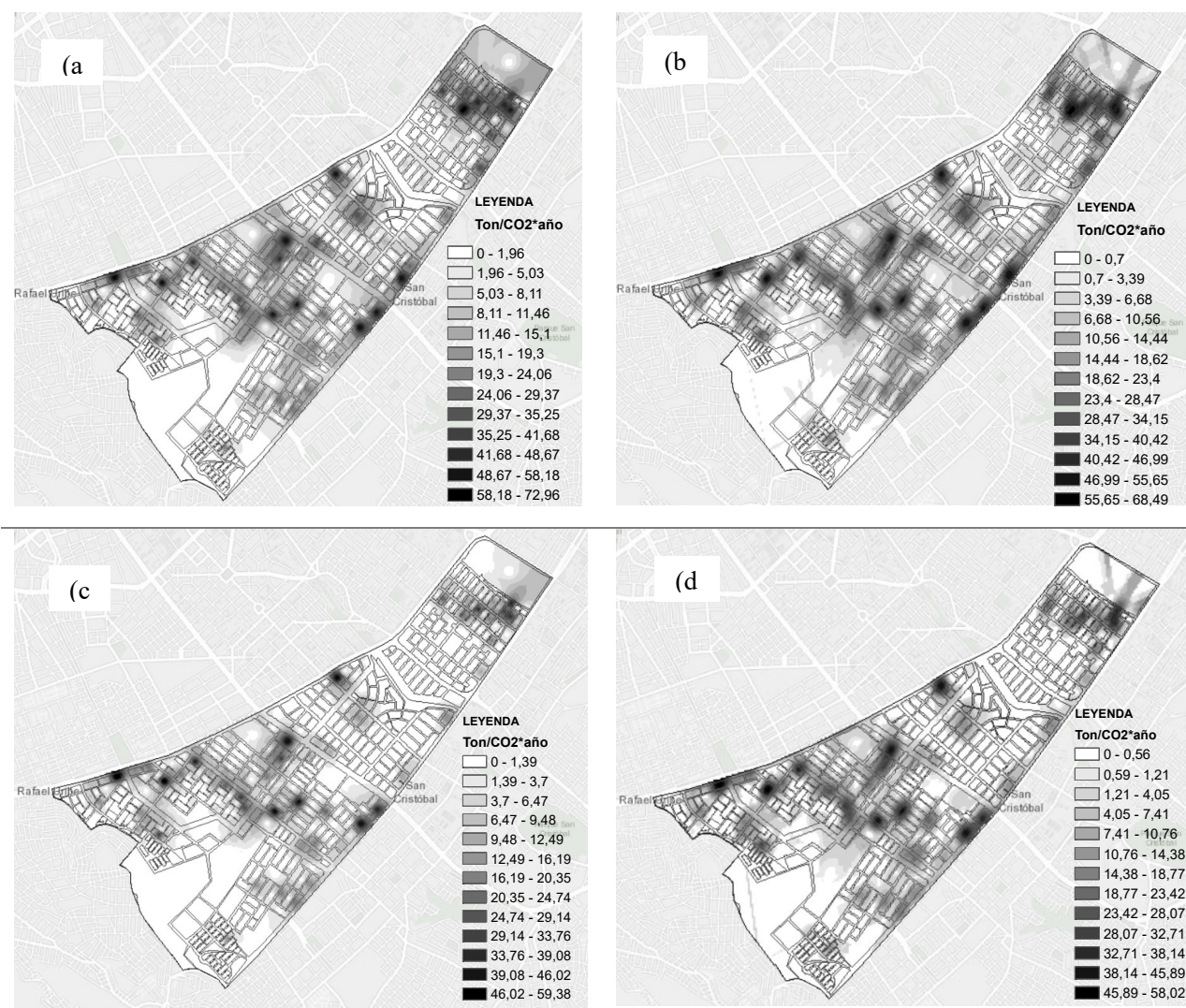
Figura 6. Resultados de la interpolación de huella de carbono actual y proyectada con la implementación de un sistema fotovoltaico para la UPZ 35 y 36 (a) Huella de carbono actual (IDW), (b) Huella de carbono actual (KRIGING), (c) Huella de carbono proyectada (IDW), (d) Huella de carbono proyectada (KRIGING)
