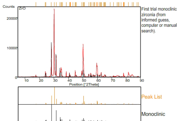
Figura 5. Difractograma, disponible en el sitio DoItPOMS para la enseñanza de la Difracción de Rayos X. Fuente: [16]
